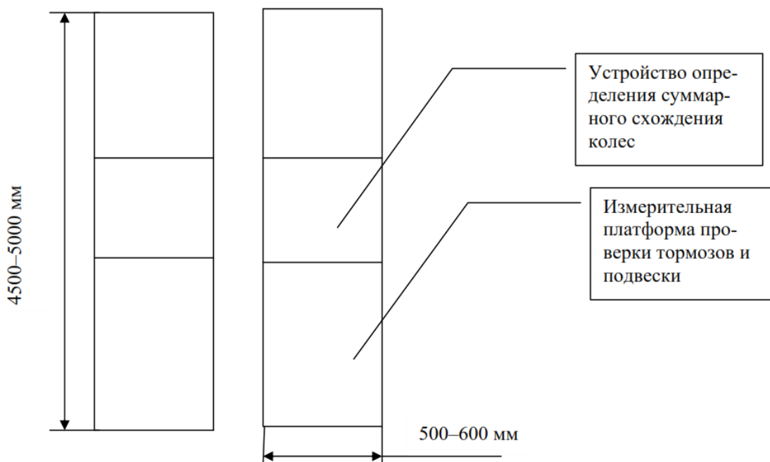
Рис. 3. Инерционный площадочный тормозной стенд
