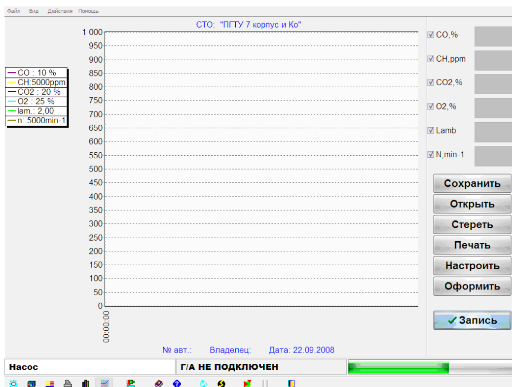
Рис. 11. Окно отображения графиков.
