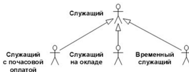
Рисунок 2.6 Пример связи обобщения
