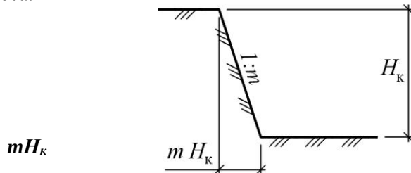
Рис. 3. Схема откоса
