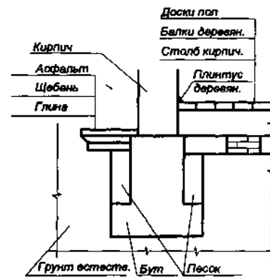
Разрез фундамента
