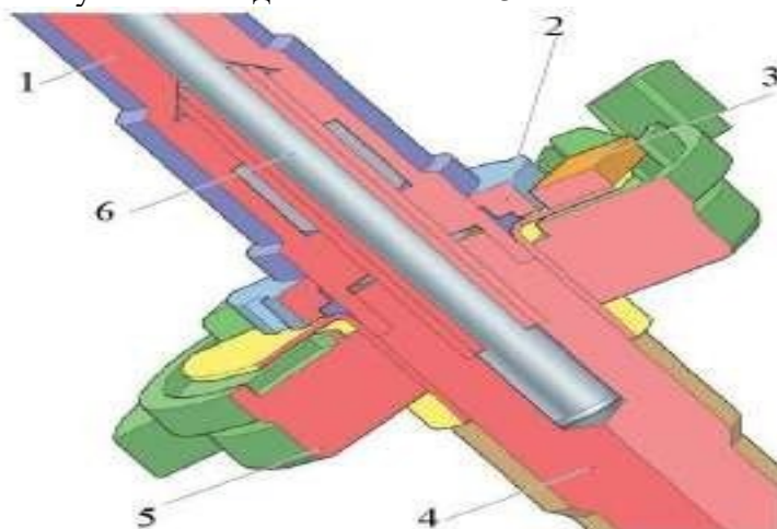
Рис. Датчик момента на рулевом колесе: 1 – рулевой вал; 2 – магнитное кольцо; 3 – чувствительный элемент датчика; 4 – вал шестерни; 5 – витой кабель; 6 – торсион
