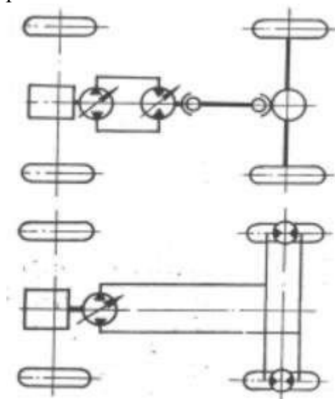
Рис. 9. Схема гидрообъемной трансмиссии: а – моноблочная, б – с отдельным расположением гидроагрегатов
