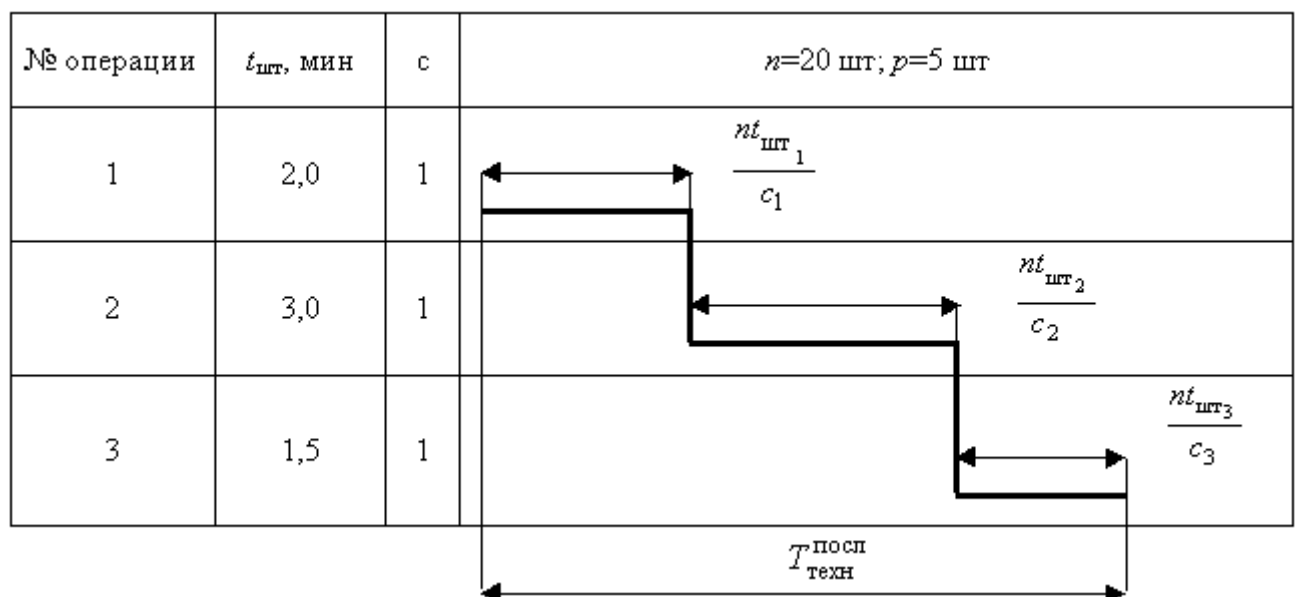
Рис.1. График технологического цикла при последовательном виде движения партии деталей в производстве
