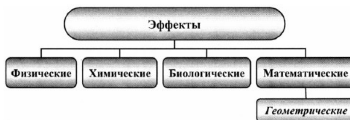
Рис.3. Классификация эффектов
