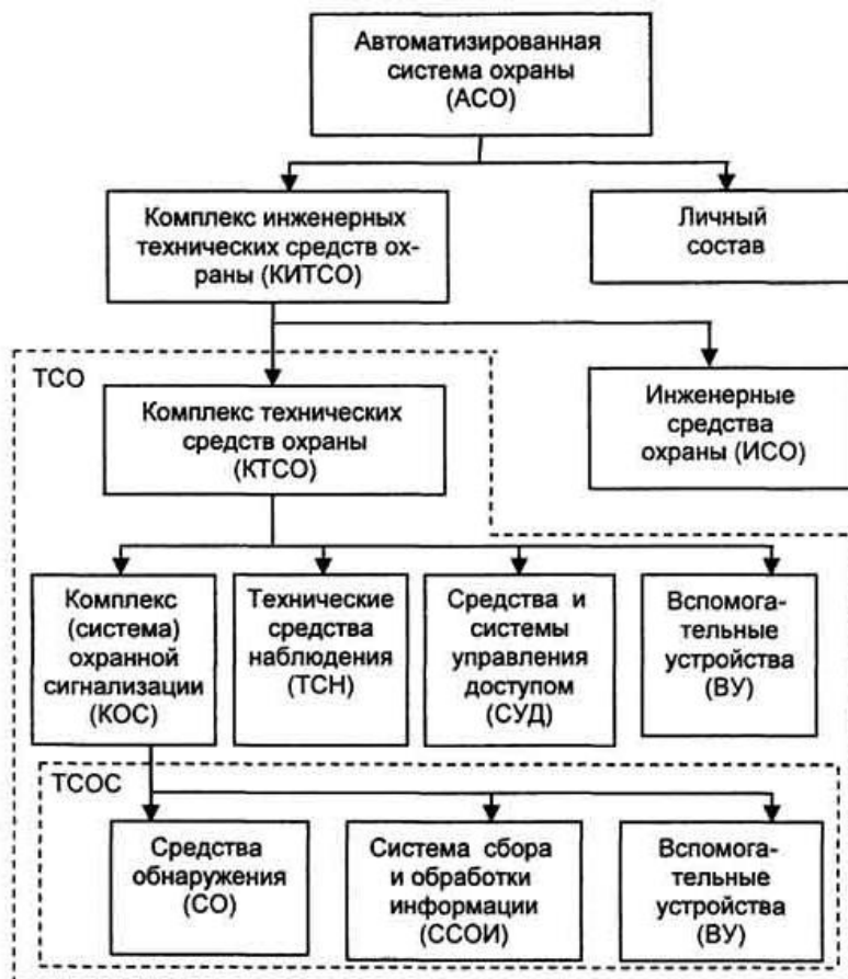
Рис. 1. Структура автоматизированной системы охраны
