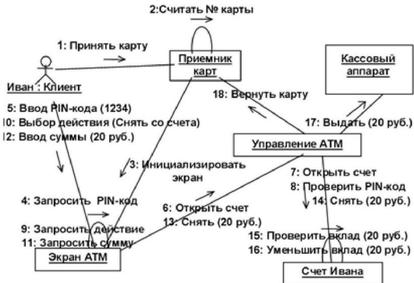
Рис. 8. Пример диаграммы кооперации
