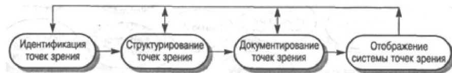
Рис. 3. Метод VORD
