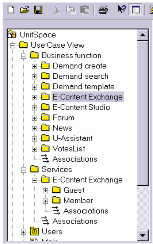
Рисунок 3 - Список бизнес-функций
