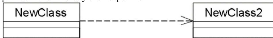
Рис. 11. Связь зависимость
