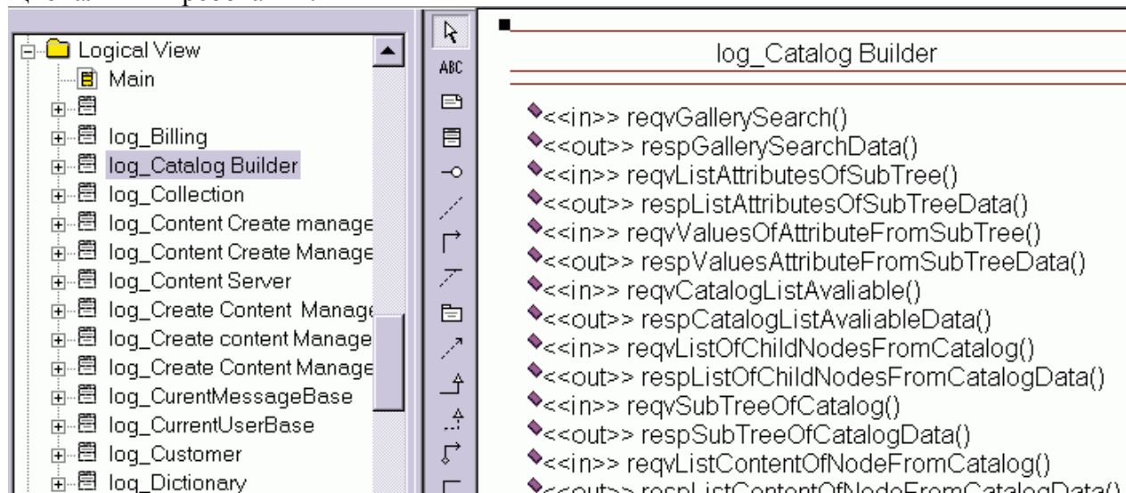
Рисунок 5 - Описание интерфейса компонентов
