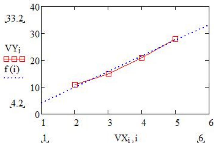
Рисунок 4.2 Линейная регрессия
