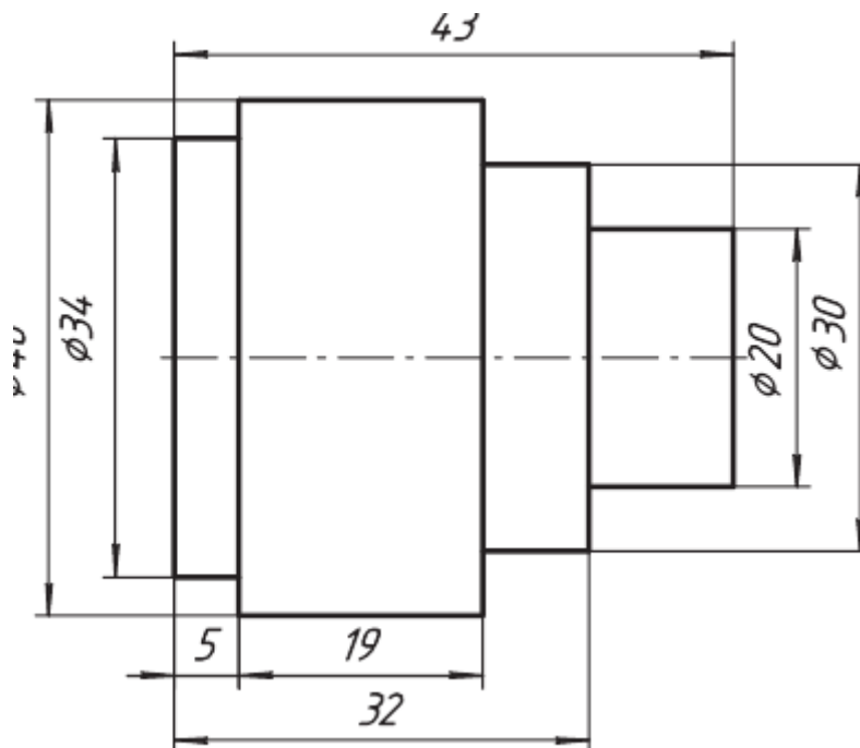
Рис. 32. Нанесение размеров
