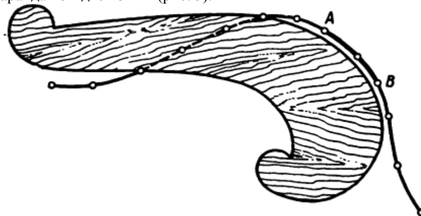
Рис. 5. Пользование лекалом
