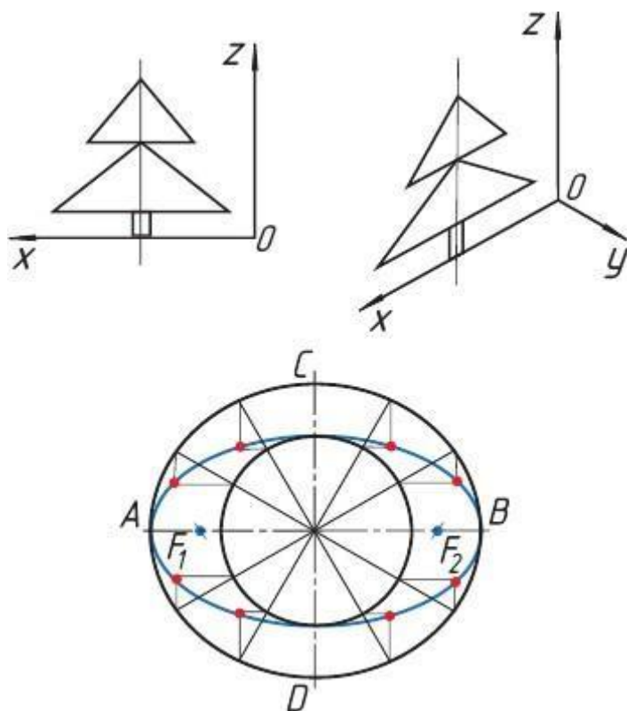
Рис. 55. Эллипс
