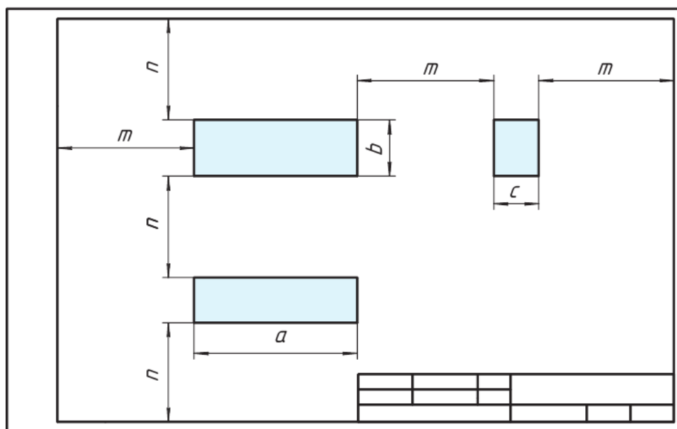
Рис. 22. Компоновка чертежа
