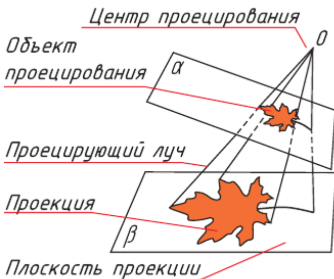
Рис. 39. Образование проекций
