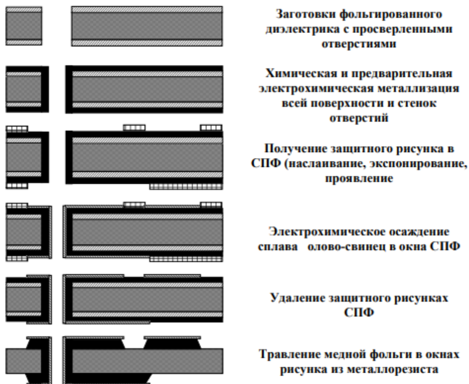
Рис.4. Изготовление ПП субтрактивным позитивным методом с использованием металлорезиста
