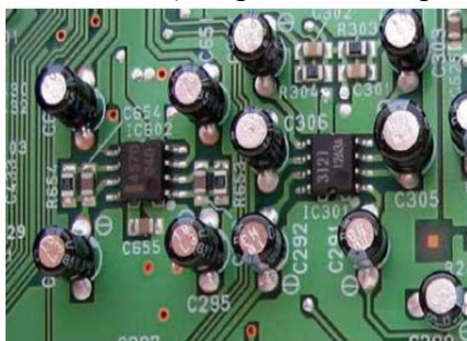
Рисунок 1 – Печатный узел
