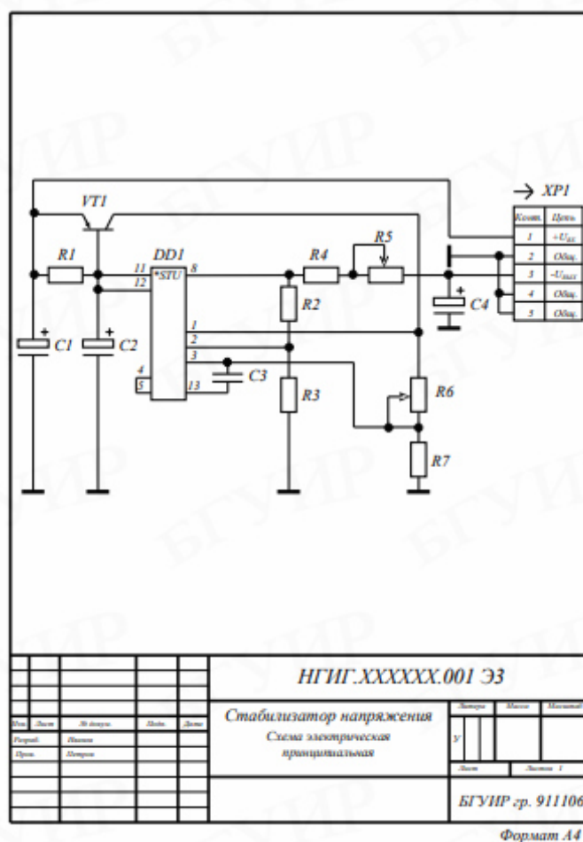
Рис.1. Схема электрическая принципиальная.
