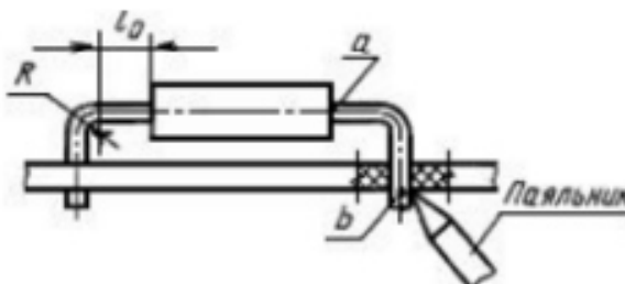
Рисунок 1 – Пример формовки ИЭТ
