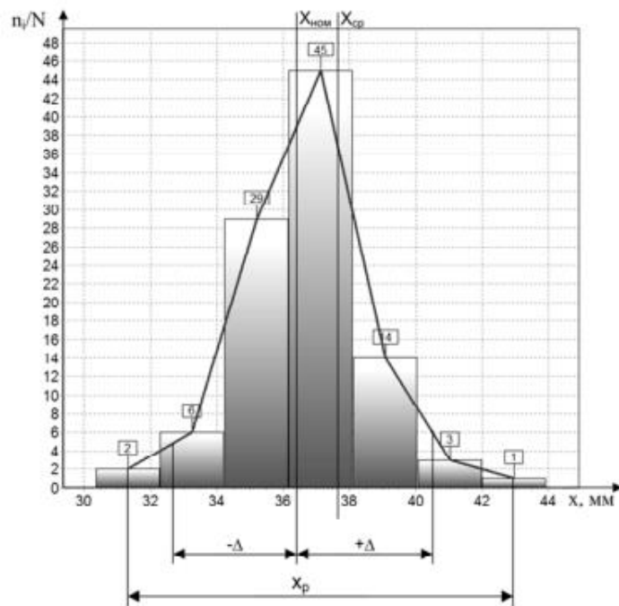
Рис. 6.2. Экспериментальная гистограмма и полигон распределения погрешностей
