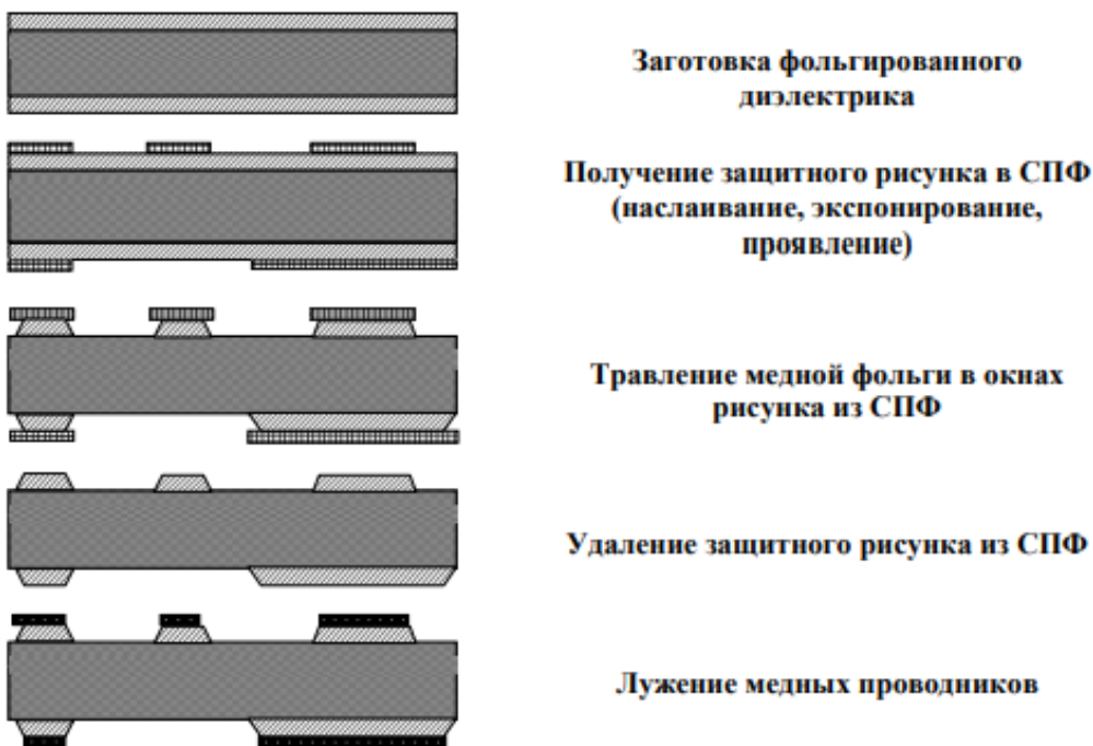
Рис.3. Изготовление ПП субтрактивным негативным методом с использованием
