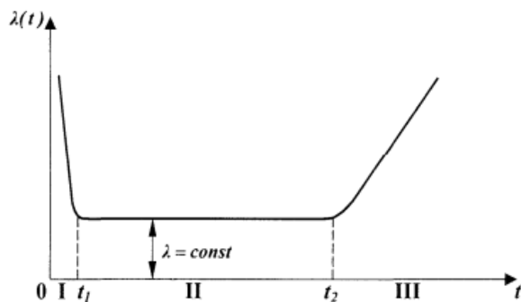
Рисунок 2 – Типичная кривая интенсивности отказов изделий от времени
