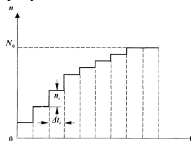
Рисунок 1 – Зависимость числа отказавших изделий от времени
