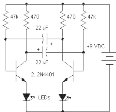
Рис.1 Схема.
