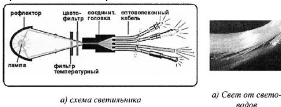
Рис. 1. Декоративный светильник из оптоволоконного
