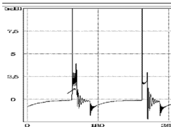
Рис. 22. Неисправность изолятора свечи
