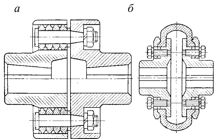
Рис.1.12. Упругие муфты
