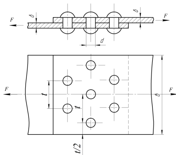
Рис. 1.16. Расчетная схема заклепочного соединения
