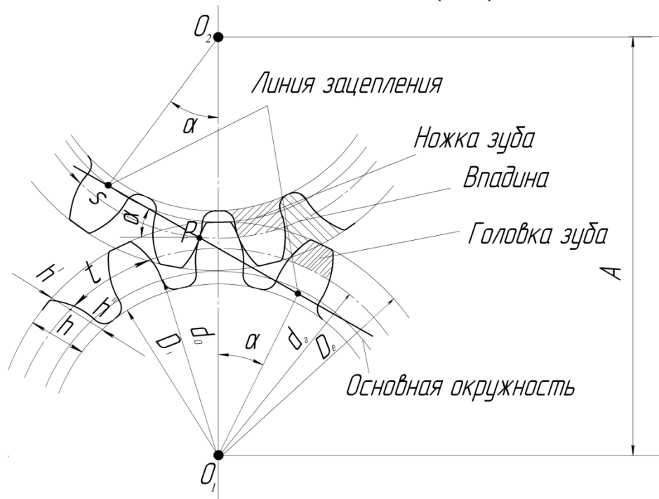
Рис. 1.5 Схема зубчатого зацепления: A – межцентровое расстояние; \alpha – угол зацепления; P – полюс зацепления; S – толщина зуба
