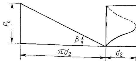
Рис. 1.19. Резьбовые соединения
