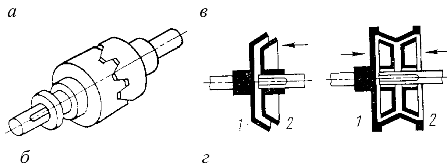
Рис. 13. Кулачковые муфты
