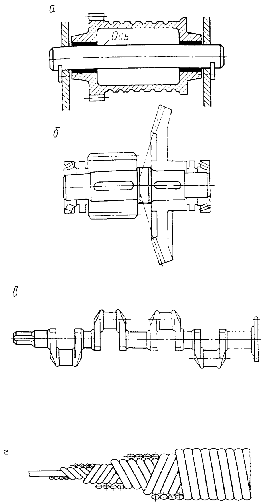
Рис. 1.7. Оси и валы
