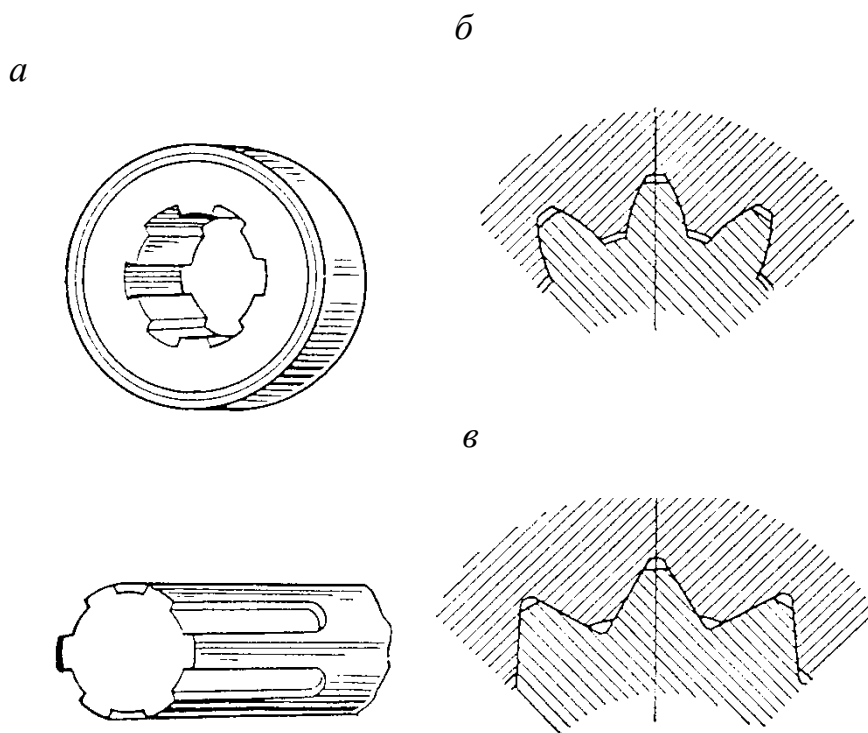
Рис. 1.27. Зубчатые соединения
