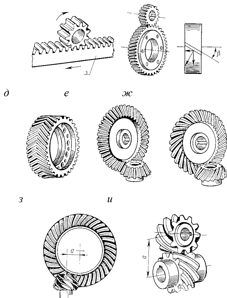
Рис. 1.4 Виды зубчатых передач: 1 – шестерня; 2 – колесо; 3 – рейка
