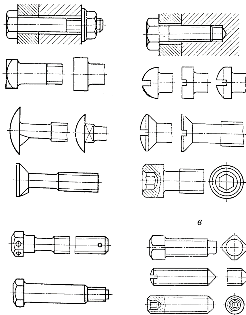
Рис. 1.20. Виды болтов и винтов
