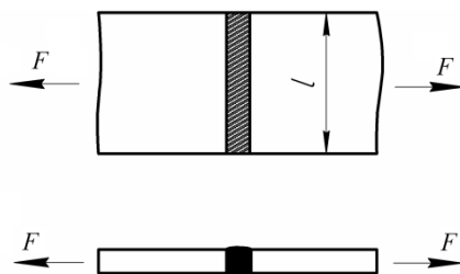
Рис. 1.18. Расчетная схема сварного соединения встык
