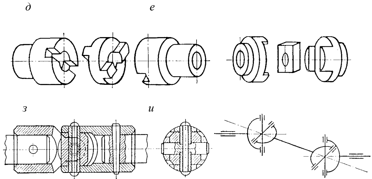
Рис. 1.11. Жесткие и компенсирующие
