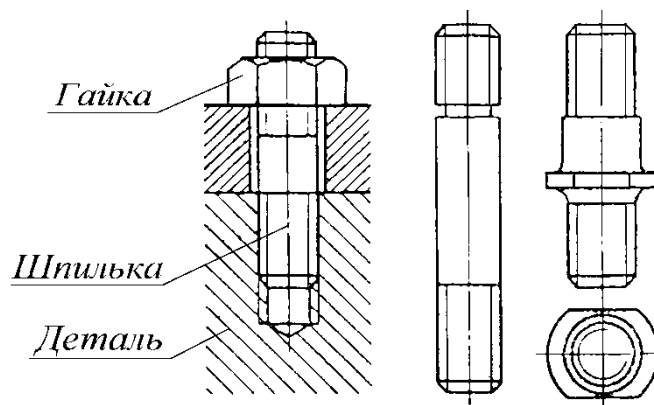
Рис. 1.21. Шпильки
