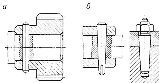
Рис. 26. Штифтовые соединения
