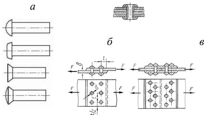
Рис. 1.15 Заклепки и заклепочные соединения
