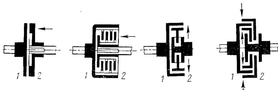
Рис. 14. Сцепные муфты
