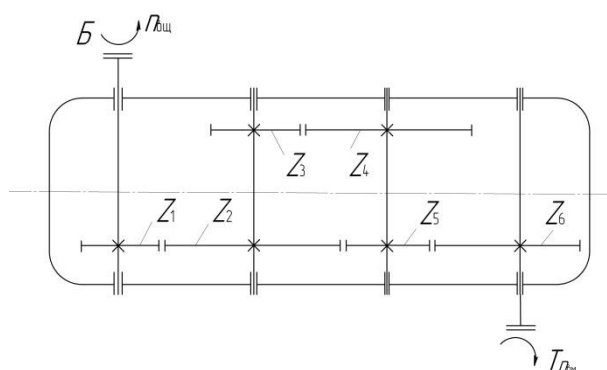
Рис. 1.6. Кинематическая схема 3 – ступенчатой зубчатой передачи (редуктора)
