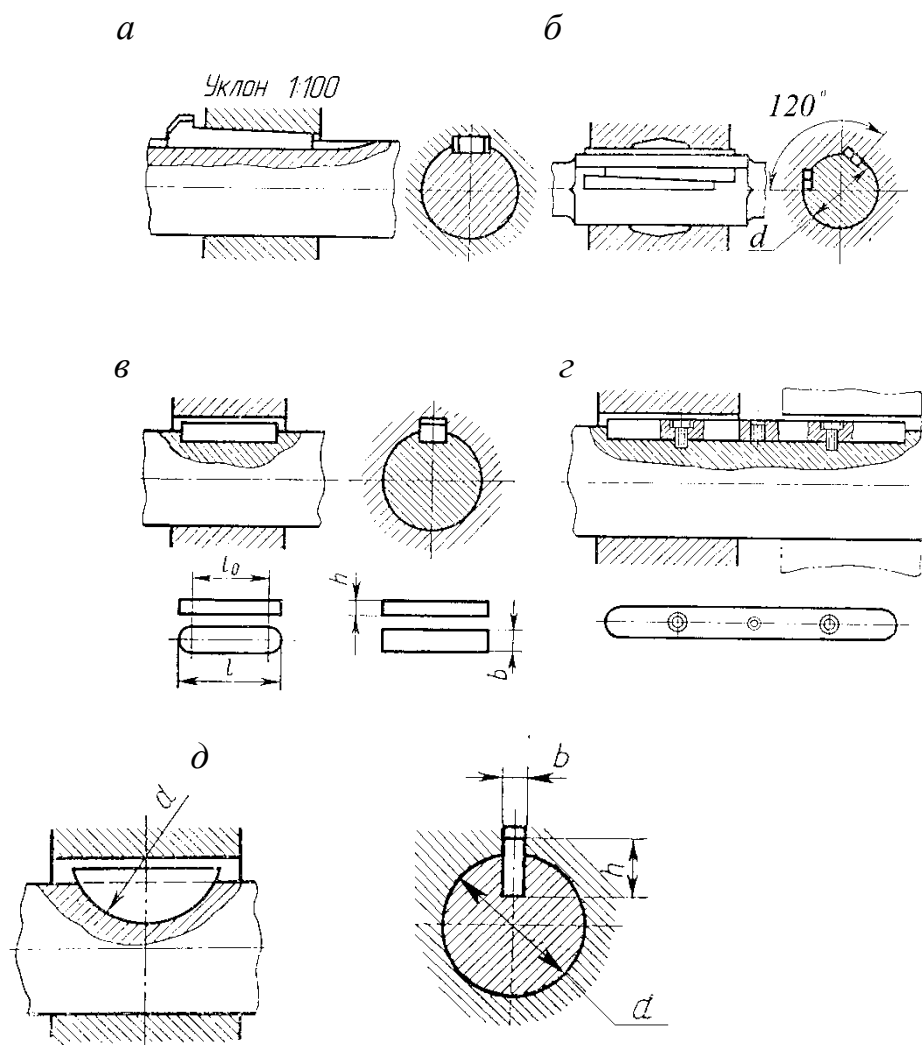
Рис. 1.25. Шпоночные соединения
