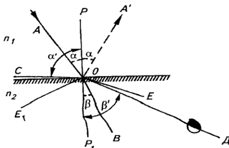
Рисунок 1 – Схема преломления лучей света
