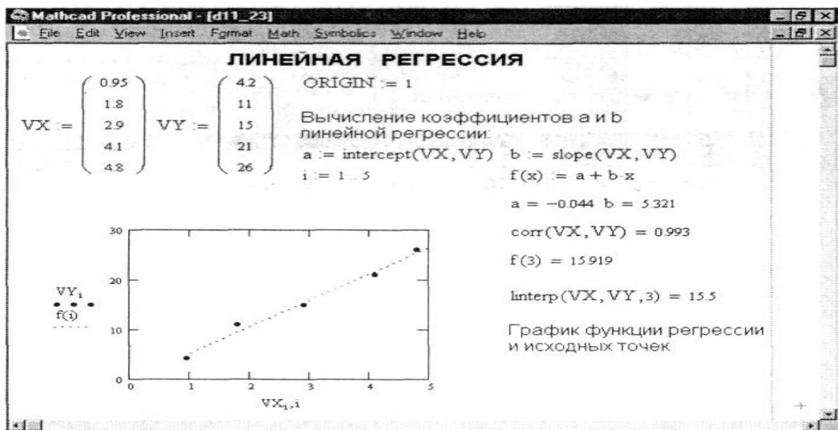
Рисунок 2 – Линейная регрессия
