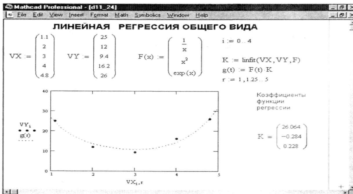
Рисунок 3 – Пример проведения линейной регрессии общего вида
