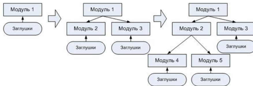
Рис. 2. Постепенная интеграция модулей при нисходящем методе тестирования
