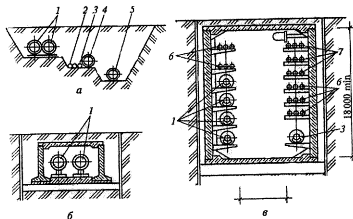
Рис. 2. Способы размещения инженерных сетей: а) в общей траншее; б) в непроходном коллекторе; в) в проходном коллекторе;
