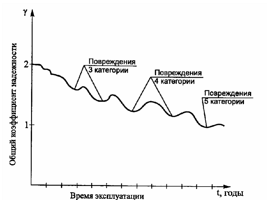
Рисунок 13.1 – Изменение надежности сооружений со временем
