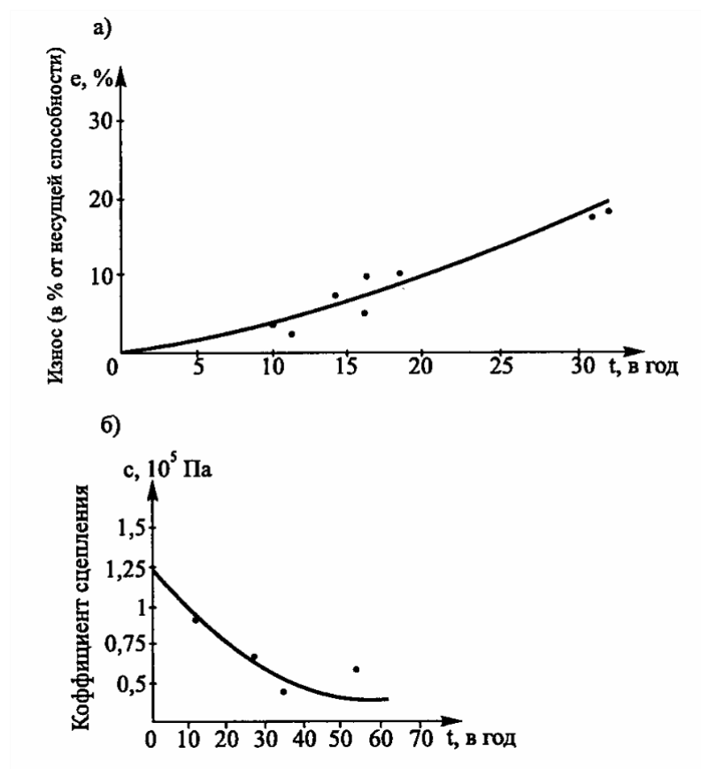
Рисунок 12.1 – Изменение надежности сооружений со временем: а – снижение несущей способности железобетонных эстакад; б – снижение сцепления глинистых грунтов в
