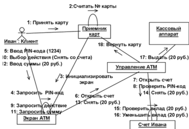
Рисунок 3.8 - Пример диаграммы кооперации
