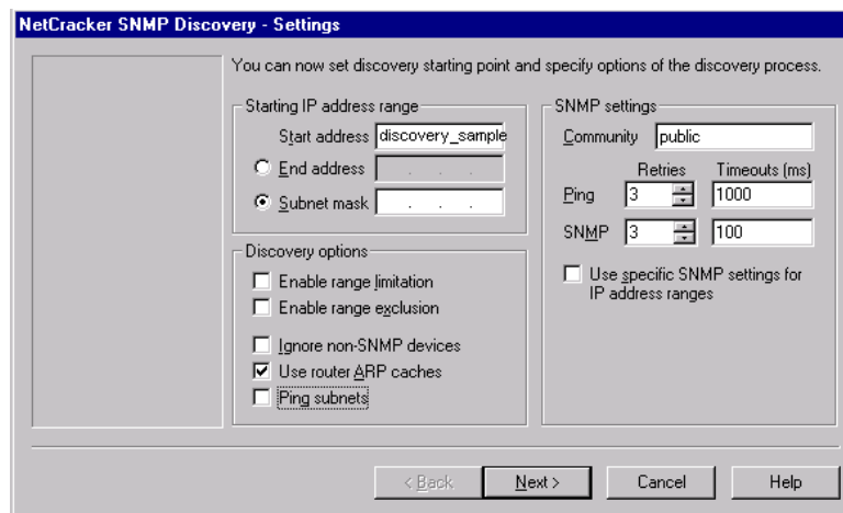
Рисунок 9.2 - Напечатать “discovery_sample” в поле start address
