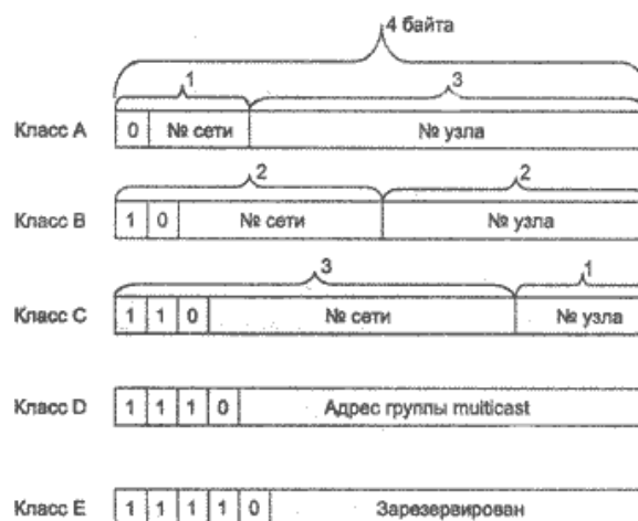
Рисунок 1.1 - Классы IP-адресов
