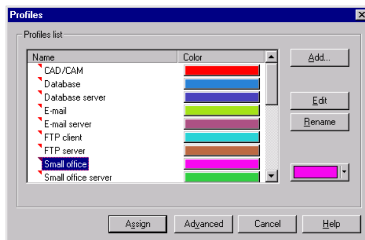
Рисунок 5.3 - Диалог конфигурации
