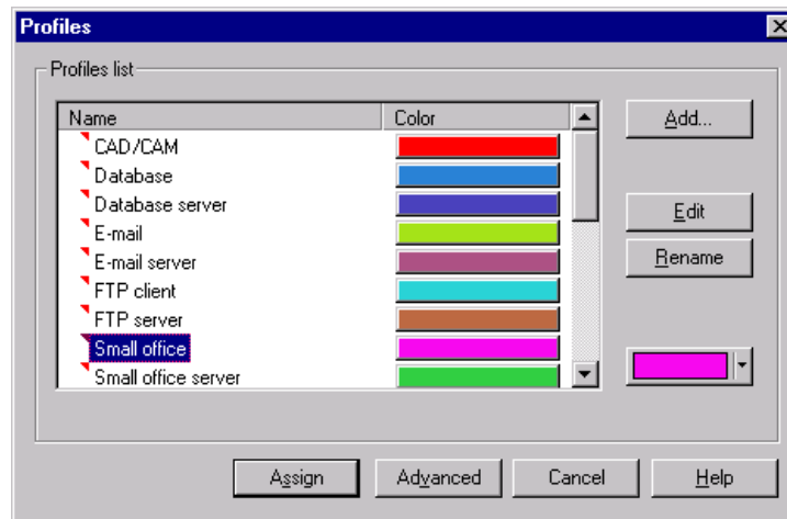
Рисунок 5.3 - Диалог конфигурации
