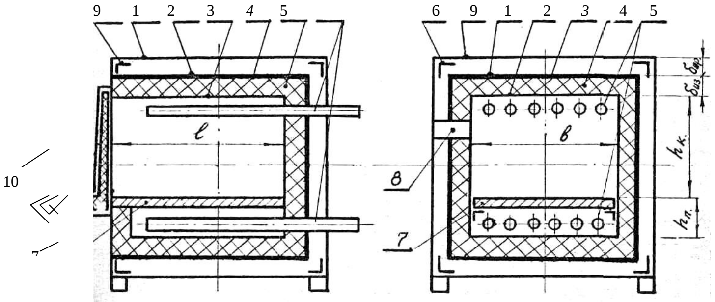
Рисунок 9.7 - Схематический разрез пекарного шкафа.
