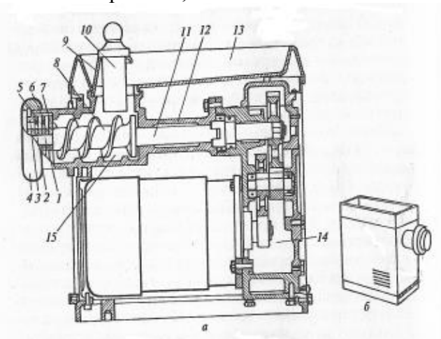
Рисунок 3.1 - Мясорубка МИМ-300
