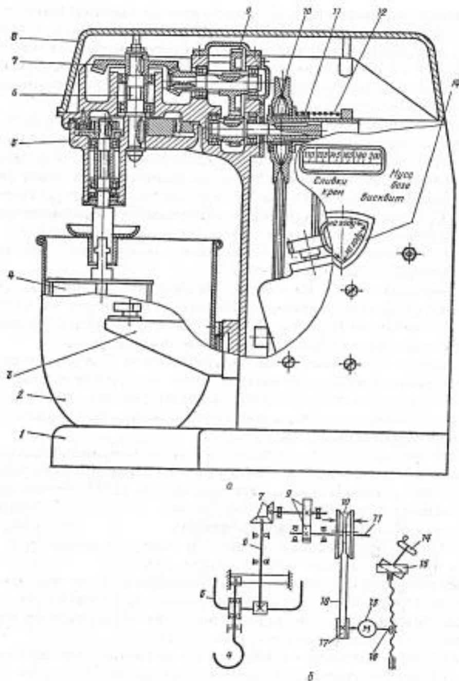
Рисунок 4.1 - Вибивальная машина МВ-6:
