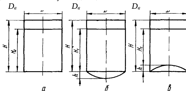
Рисунок 7.4 - Конфигурация варочных сосудов:
