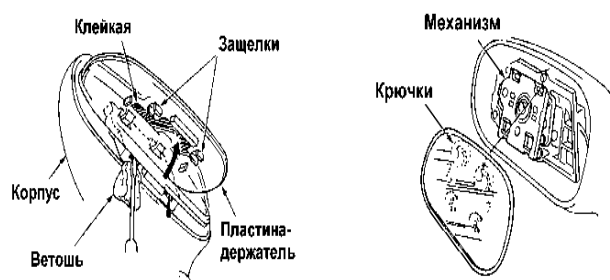
Рис. 4.1. Снятие пластины Рис. 4.2. После снятия пластины
