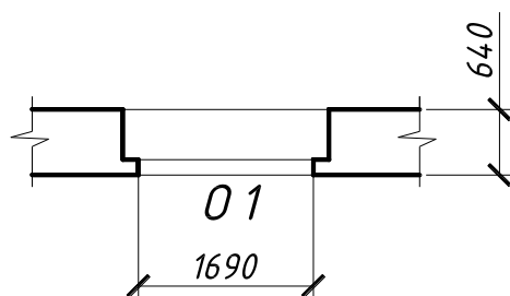
Рисунок 10 - Оконный проем
