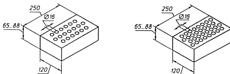
Рис. 1. Керамический кирпич– пустотелый а) с 19 , б) с 32 пустотами
