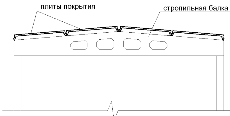
беспрогонный вариант покрытия
