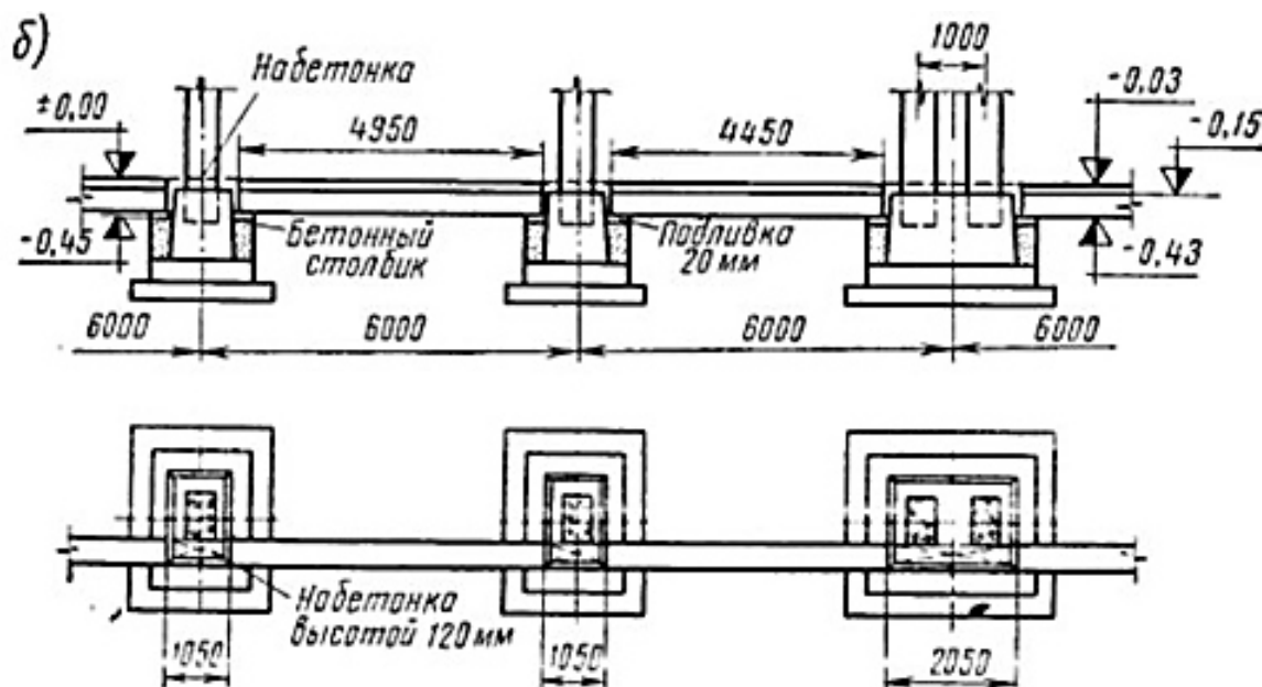
Рисунок 4. Укладка фундаментных балок
