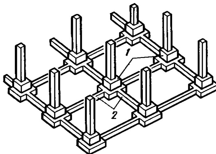
Рис. 30.4. Схема столбчатых фундаментов с антисейсмическими связями:
