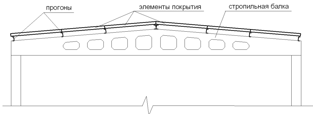
прогонный вариант покрытия
