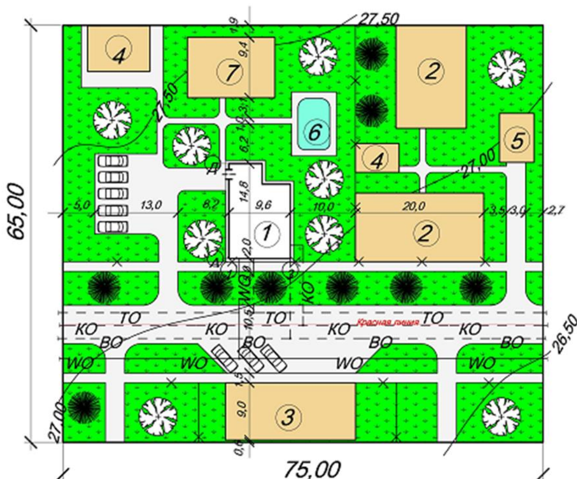
Рисунок 1 Генплан М 1:500
