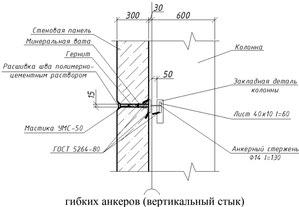
Рисунок 2- узел крепления стеновой панели к колонне каркаса при помощи гибких анкеров (горизонтальный стык)
