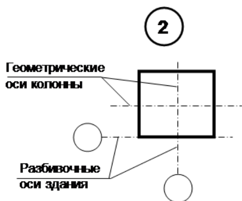
Рис. 3.4. Нулевая привязка
