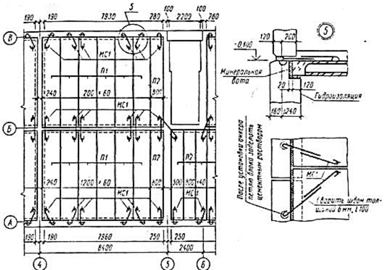
Спецификация изделий к плану перекрытия
