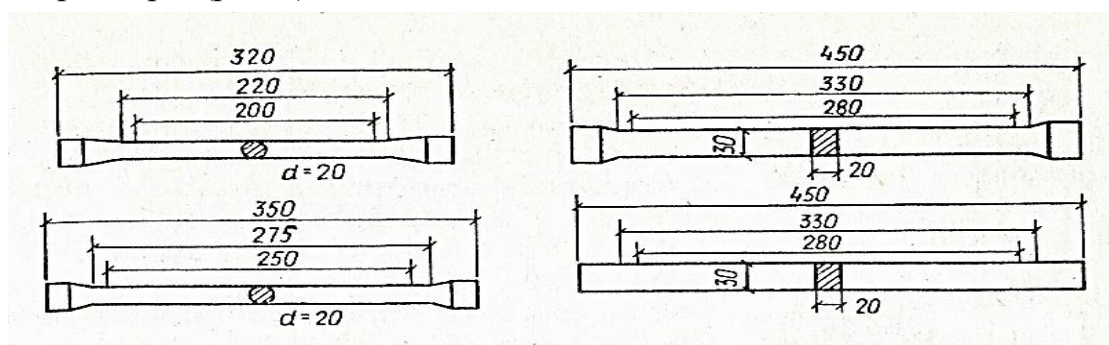
Рис 1. Образцы стали для испытания на растяжение.
