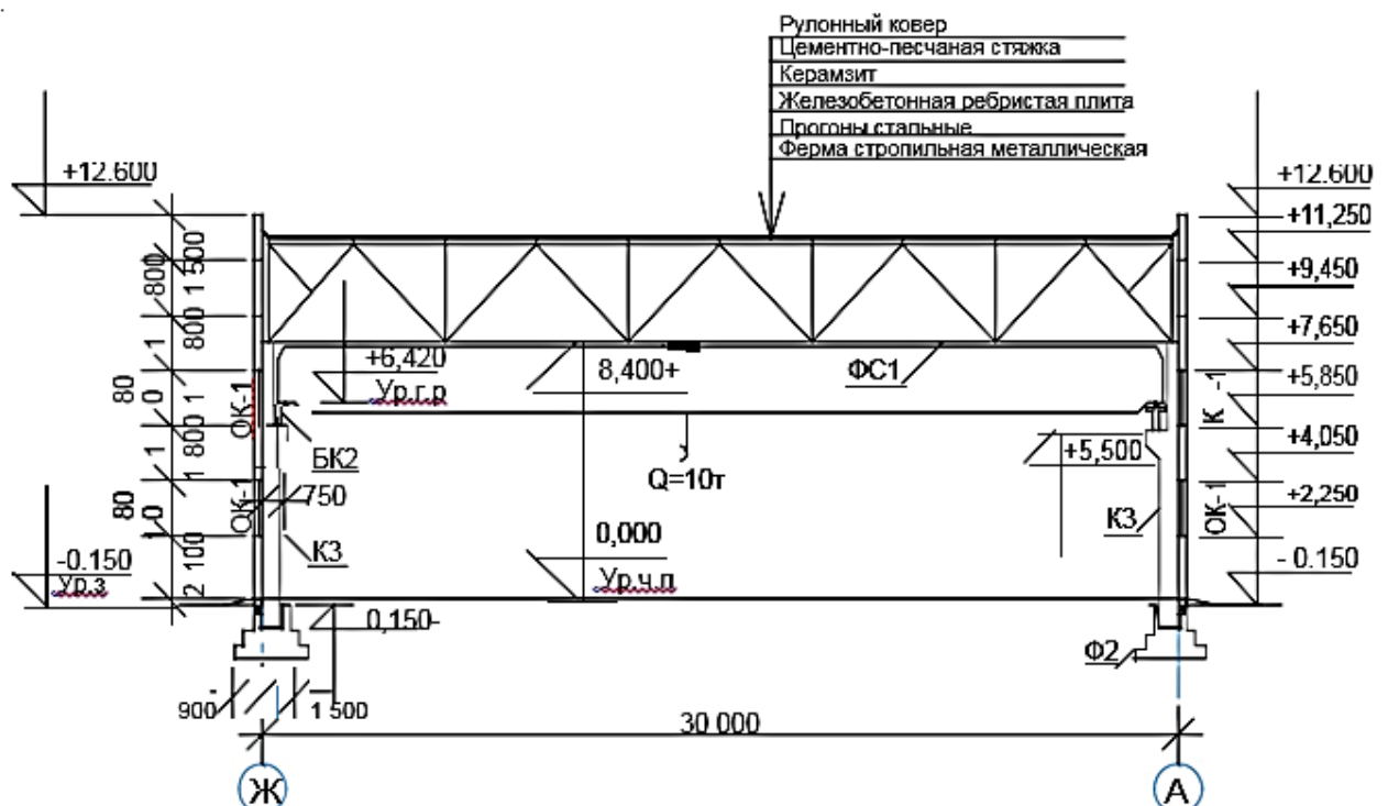
Рисунок 1. Поперечный разрез промышленного здания
