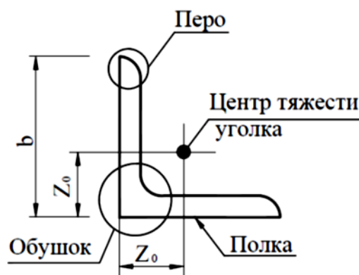
Рисунок1. Профили стального проката
