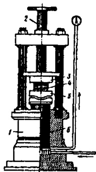
Схема гидравлического пресса для испытания на сжатие: 1 - станина; 2 - винтовое приспособление для зажима образца; 3 - верхняя опорная плита; 4 - испытуемый образец; 5 - нижняя опорная плита с шаровой поверхностью; 6 - поршень
