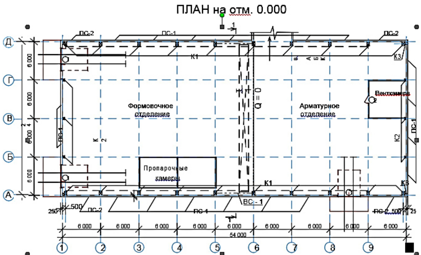
Рисунок 2. Пример выполнения плана промышленного здания
