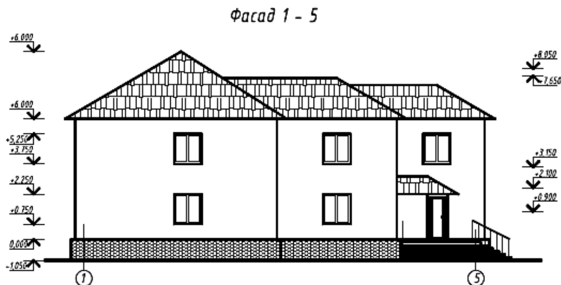
Рис.1 Образец выполнения фасада здания
