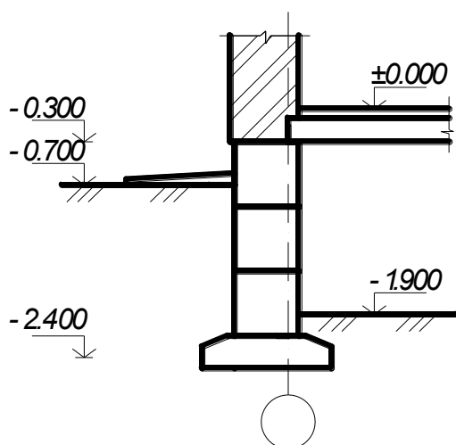
Рисунок 8 - Определение высоты фундамента
