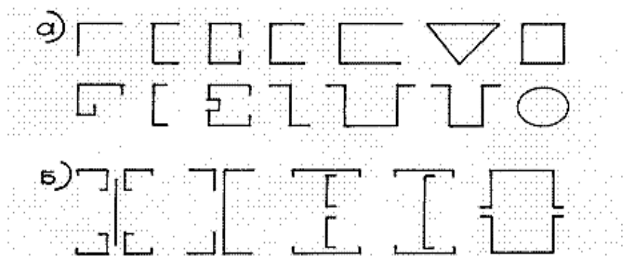
Рис. 2.2. Сортаменты холодногнутых профилей:
