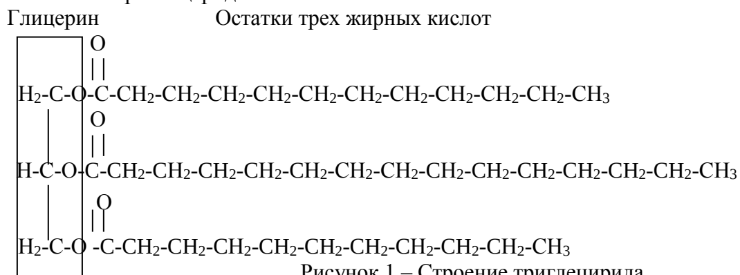
Рисунок 1 – Строение триглицерида
