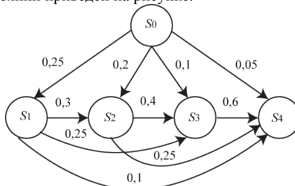
Размеченный граф состояний четырех объектов
