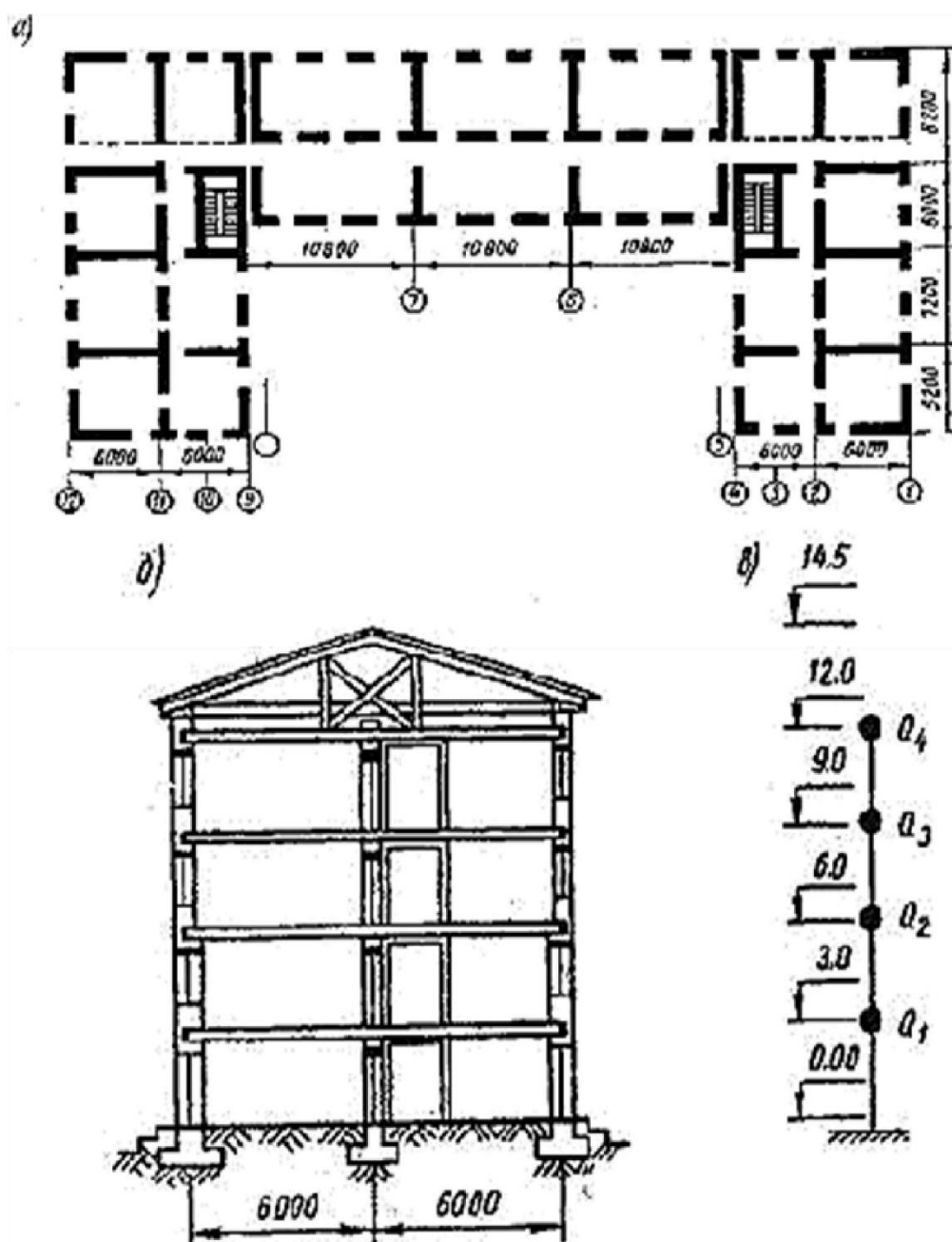
Рисунок 5.1 – Кирпичный жилой дом: а – план типового этажа; б – поперечный разрез (перегородки условно не показаны); в – расчетная схема
