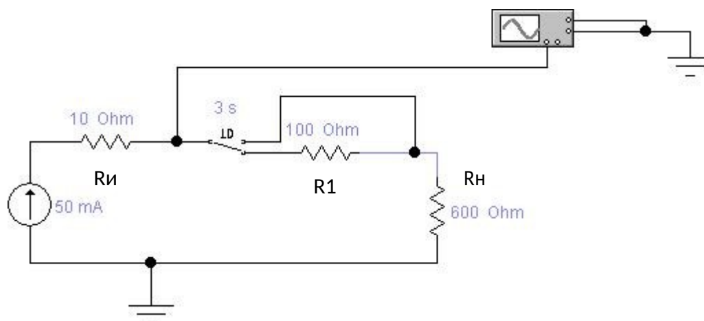
Рисунок 15 – Эквивалентная схема 1 замещения работы кабельного радара
