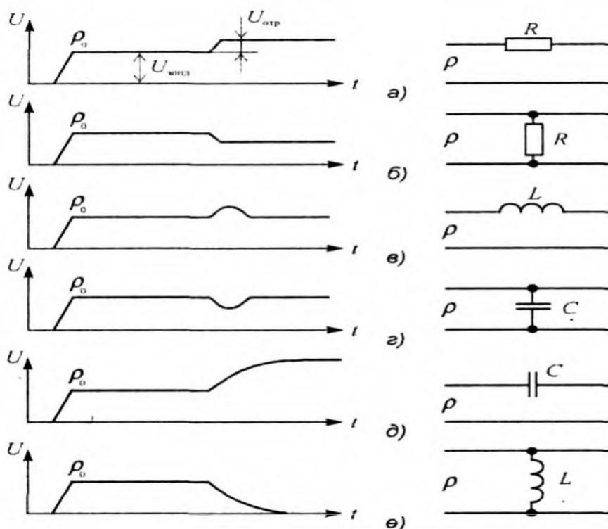
Рисунок 11 – Рефлектограммы простейшей неоднородности:
