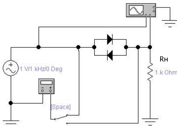
Рисунок 4 – Эквивалентная схема замещения диодного ограничителя
