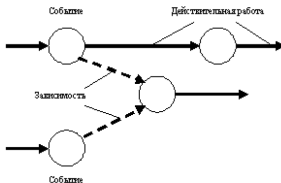
Рис. 1 Основные элементы сетевой модели
