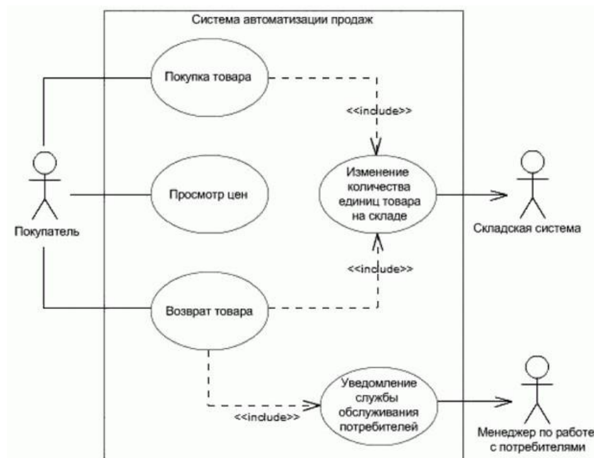
Рис. 1 Пример диаграммы прецедентов
