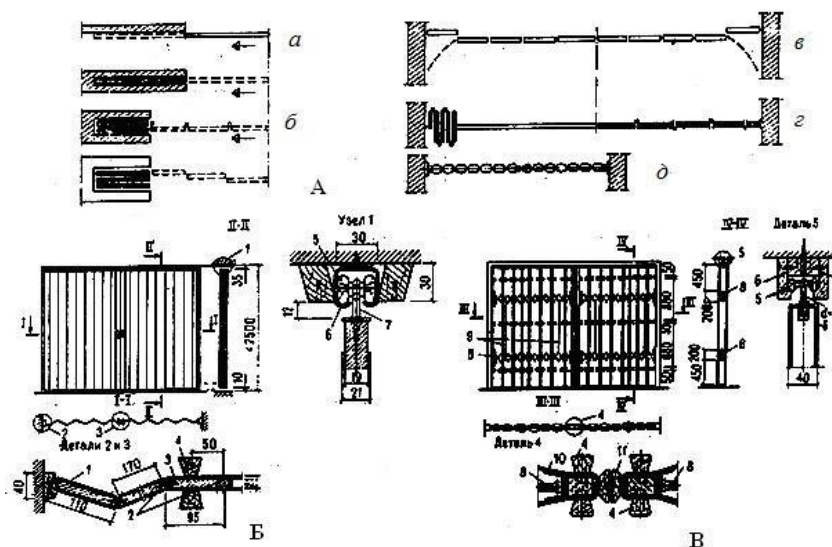
Рис. 47. Трансформируемые перегородки:
