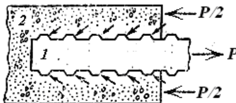
Рис. 64. Сцепление арматуры с бетоном: 1 — арматура периодического профиля; 2 — затвердевший бетон
