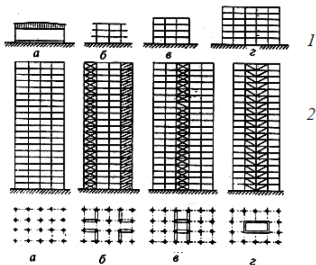
Рис. 20. Каркасы:
