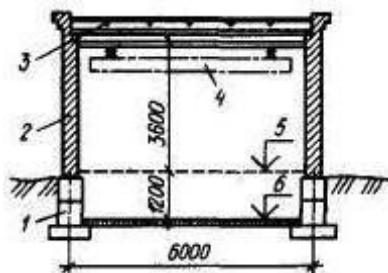
Рис. 111. Конструктивная схема унифицированного здания систем водоснабжения и канализации при пролете 6:
