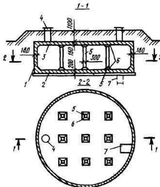
Рис. 118. Конструктивное решение круглого монолитного резервуара: 1 — стенка резервуара; 2 — днище; 3 — перекрытие; 4 — люк; 5 — колонна; 6 — капитель колонны; 7 — приямок
