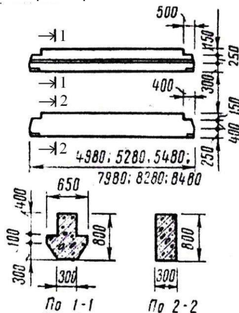
Рис. 103. Железобетонные ригели многоэтажных промзданий
