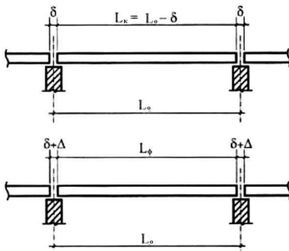
Рис. 1. Размеры конструктивного элемента: L_o — модульный; L_n — конструктивный; L_\phi — фактический
