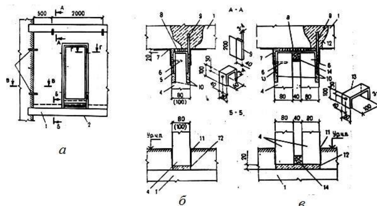
Рис. 45. Перегородки из гипсобетонных панелей и их крепления к несущим конструкциям:
