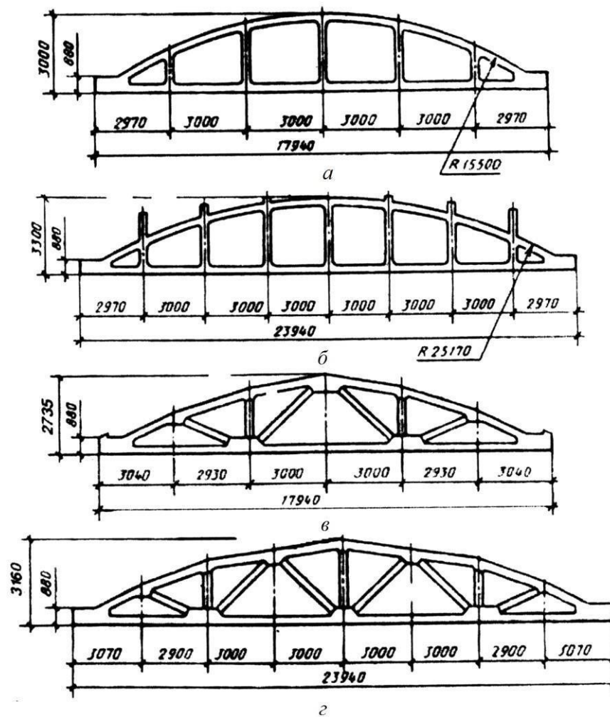
Рис. 73. Железобетонные фермы: a — арочная сегментная безраскосная ферма пролетом 18 м; б — то же, пролетом 24 м; в — сегментарная раскосная ферма пролетом 18 м; г — то же, пролетом 24 м
