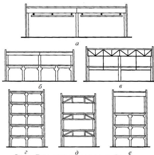
Рис. 86. Производственные здания различной этажности:
