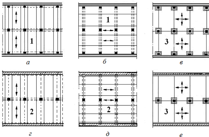
Рис. 6 Конструктивные схемы каркасных зданий:
