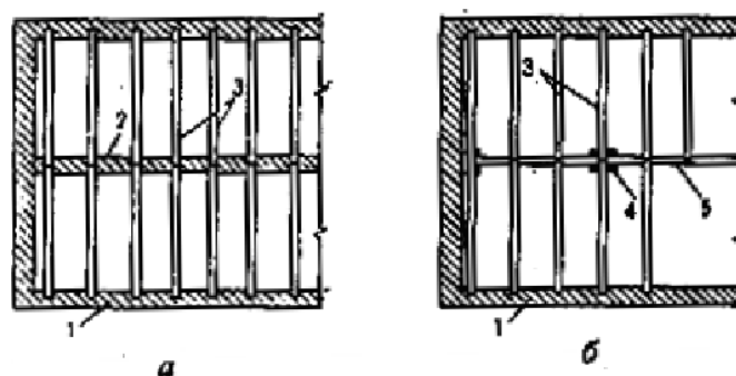
Рис. 35. Расположение балок перекрытия:
