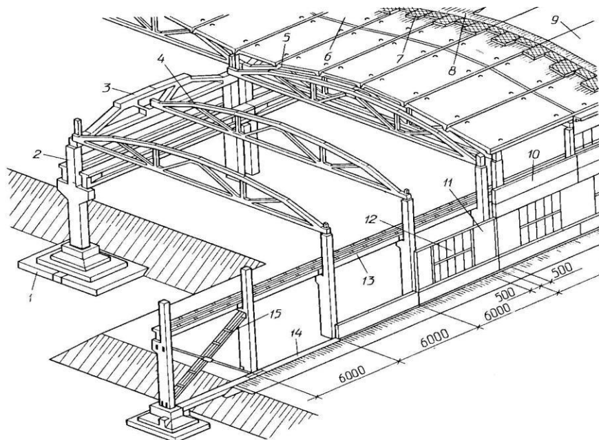
Рис. 87. Железобетонный каркас одноэтажного промзданиясо стропильными и подстропильными фермами:
