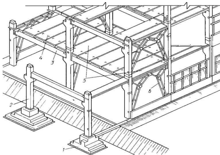
Рис. 101. Железобетонный каркас многоэтажного промышленного здания: 1 — фундамент; 2 — колонна; 3 — ригель; 4 — настил междуэтажного перекрытия; 5 — связевые плиты; 6 — вертикальные «портальные» связи
