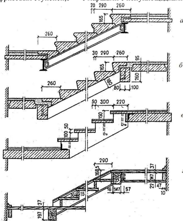
Рис. 29. Конструктивные решения лестниц из мелких элементов:
