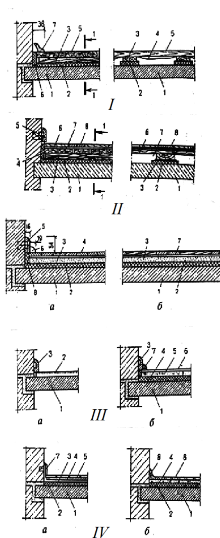
Рис. 39. Типы полов:
