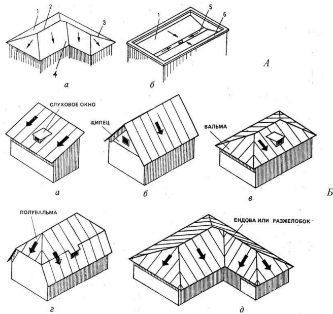
Рис. 30. Ребра и плоскости крыш, формы скатных крыш:
