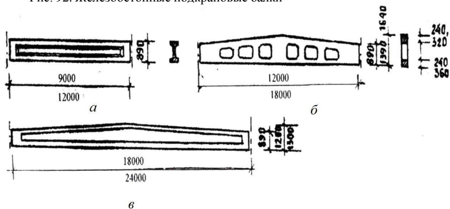
Рис. 93. Железобетонные стропильные балки: а — балка с параллельными поясами двутаврового сечения; б — полигональная балка перфорированной стенкой; в — полигональная балка двутаврового сечения
