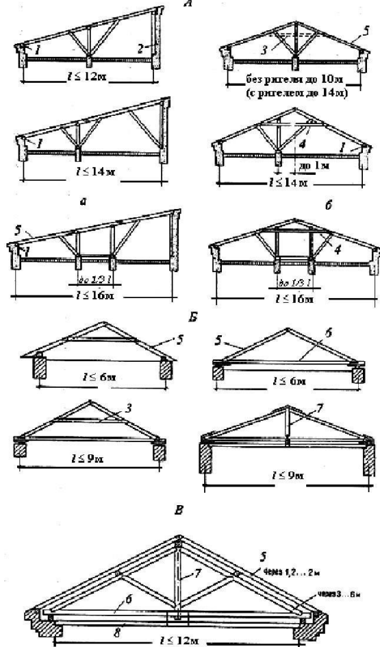
Рис. 31. Схемы деревянных несущих конструкций скатных крыш:
