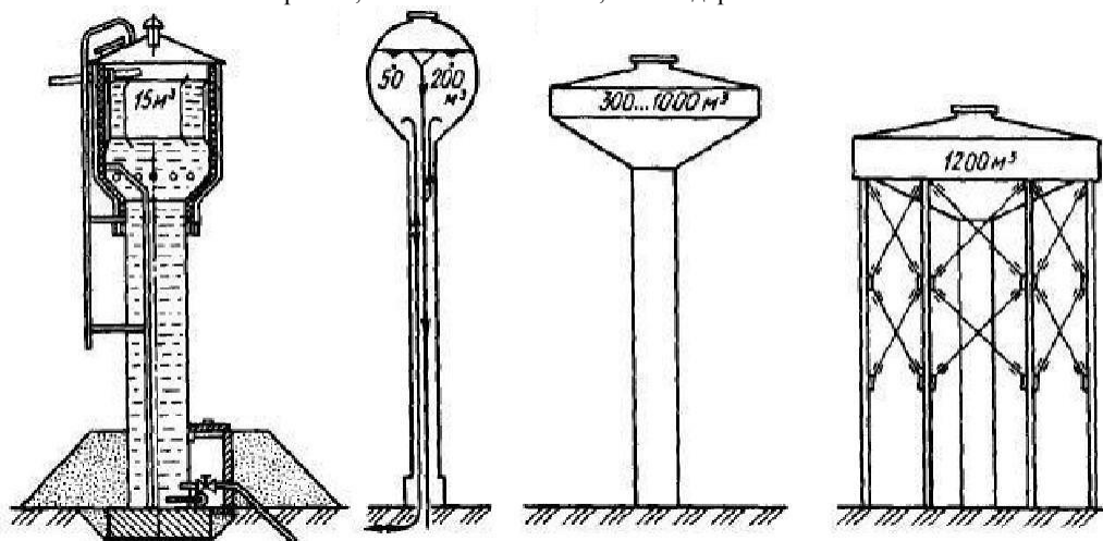
Рис. 113. Металлические водонапорные башни различного конструктивного типа
