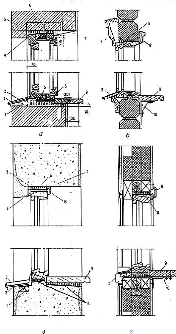
Рис. 41. Установка оконных блоков в стенах: а — кирпичных; б — деревянных брусчатых; в — панельных легкобетонных; г — панельных из листовых материалов; 1 — деревянная антисептированная пробка; 2 — стальной костыль; 3 — слив из оцинкованной стали; 4 — герметик; 5 — конопатка; 6 — рубероид; 7 — штукатурка; 8 — наличник; 9 — подоконная доска; 10 — стальная консоль
