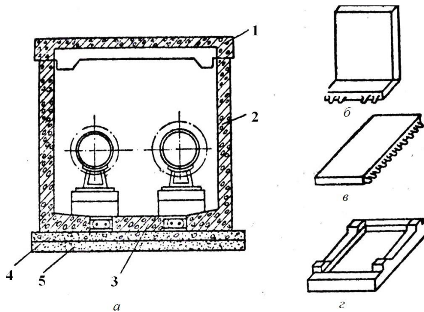
Рис. 127. Сборный полупроходной канал из железобетонных блоков: a — сечение канала; б — блок стены; в — блок днища; г — блок перекрытия; 1 — ребристый блок покрытия; 2 — стеновой блок; 3 — блок днища; 4 — бетонная подготовка; 5 — щебеночная подготовк
