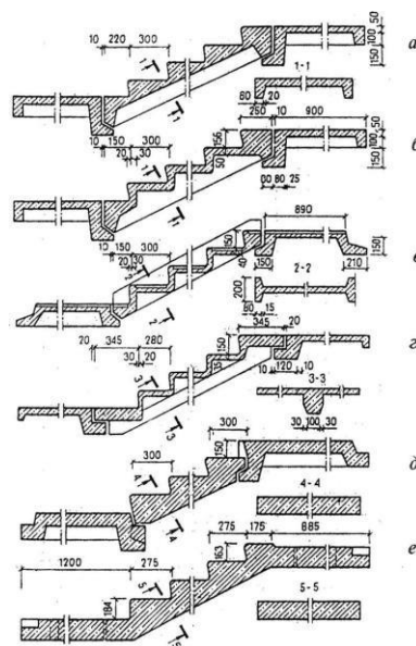
Рис. 28. Конструктивные решения железобетонных сборных лестниц из крупных элементов:
