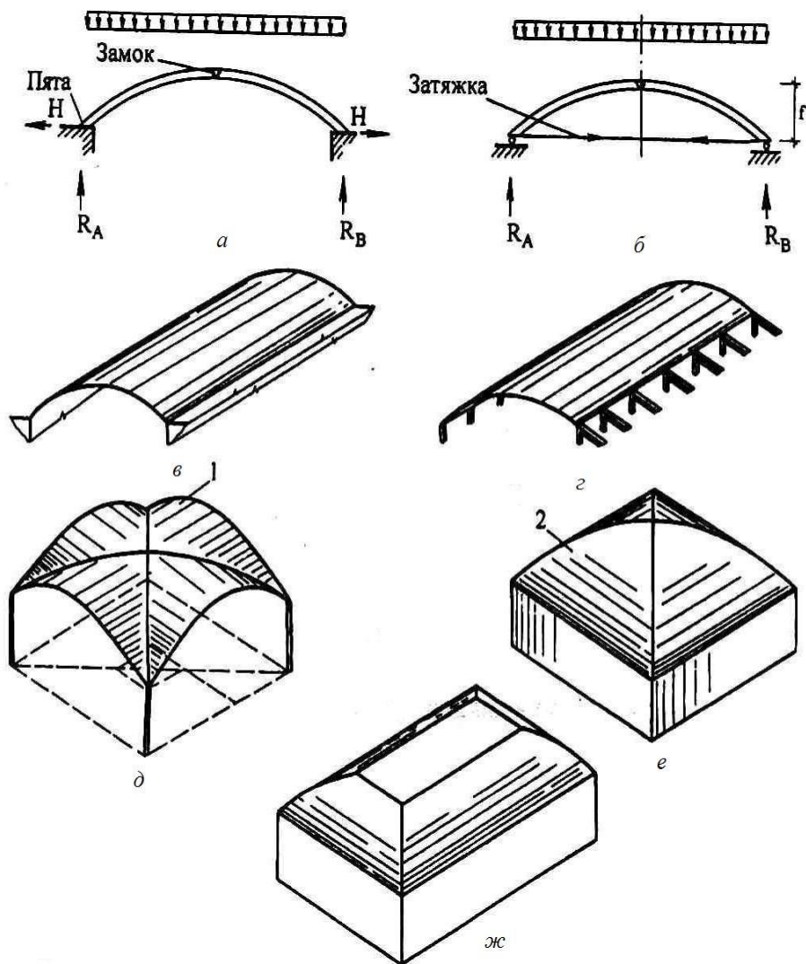
Рис. 49 Арочно-сводчатые конструкции: a — арка; б — арка с затяжкой; в — цилиндрический свод; г — цилиндрический свод на стоечно — подкосных опорах; д — крестовый свод; е — сомкнутый (монастырский) свод; ж — «зеркальный свод»; R_A и R_B — вертикальные реакции опор; H — распор; f — стрела подъема арки; 1 — распалубка; 2 — лоток
