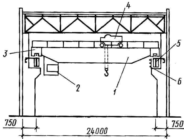
Рис. 100. Одноэтажное промздание с мостовыми кранами: 1 — опорный мост; 2 — кабинка крановщика; 3 — механизм передвижения вдолькранового пути; 4 — подъемное устройство на тележке; 5 — подкрановая балка; 6 — токопровод
