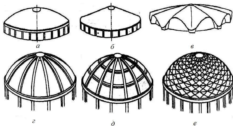
Рис. 50 Современные купольные конструкции: a, б — тонкостенные гладкие; в — волнистый купол из железобетона; г — ребристый; д — ребристо — кольцевой, е — сетчатый купол из стальных стержней
