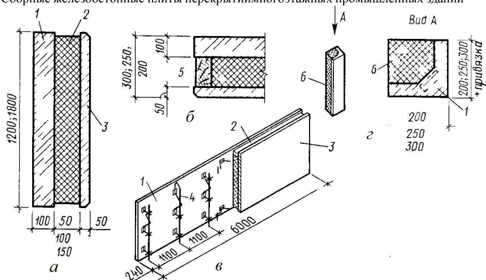
Рис. 104. Сборные железобетонные плиты перекрытий многоэтажных промышленных зданий
