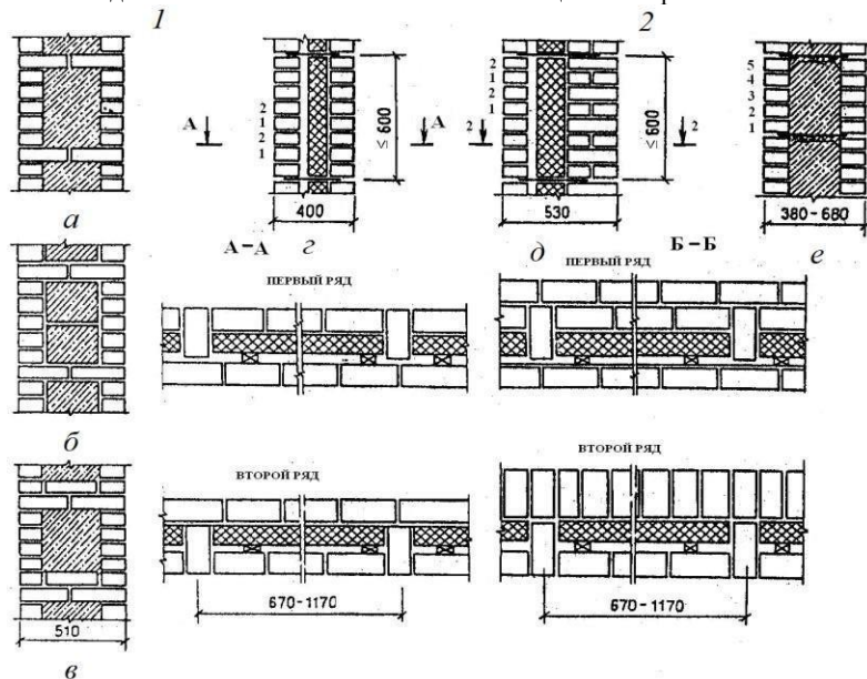
Рис. 15. Облегченные кладки многослойных наружных стен:
