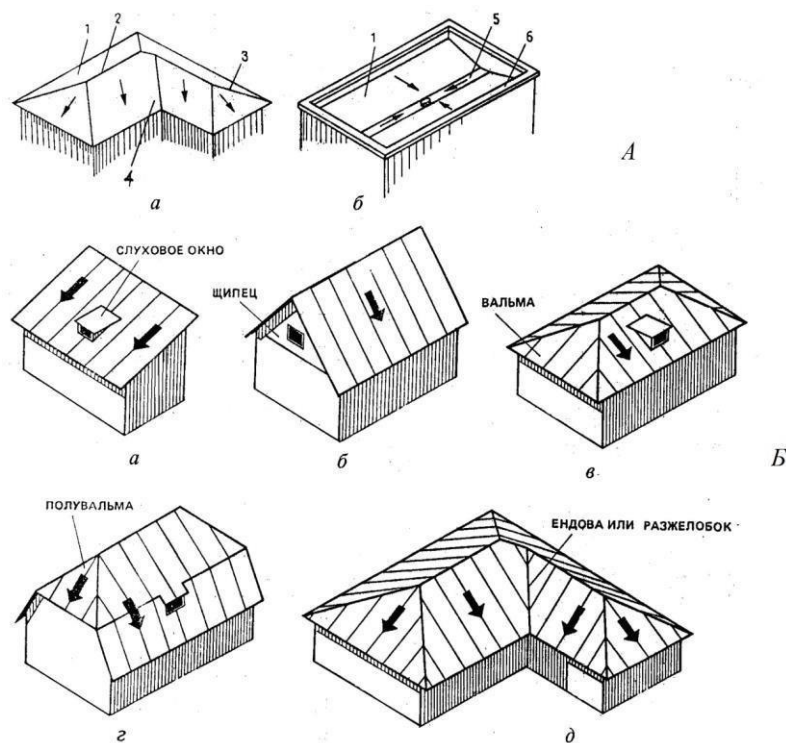
Рис. 30. Ребра и плоскости крыш, формы скатных крыш:
