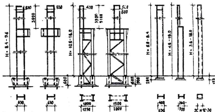
Рис. 95. Металлические колонны промышленных зданий: a — колонны постоянного сечения при мостовых кранах Q \leq 20 т; б — двухветвевые колонны при мостовых кранах Q \leq 50 т; в — колонны для бескрановых зданий и задний с подвесными кранами; г — стальные фахверковые колонны
