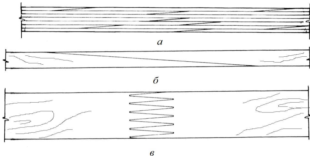
Рис. 79. Варианты клеевых соединений деревянных элементов: a — послойное клеевое соединение; б — диагональное соединение «в нахлестку»; в — зигзагообразное соединение в ус
