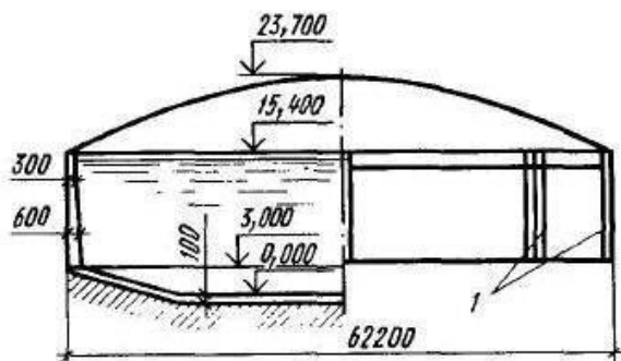
Рис. 119. Предварительно напряженный резервуар (фрагменты разреза и фронтального вида):
