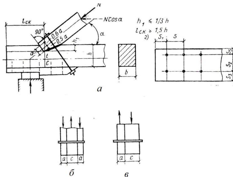
Рис. 77. Соединения элементов деревянных конструкций: a — лобовая врубка; б — симметричное нагельное соединение; в — несимметричное нагельное соединение
