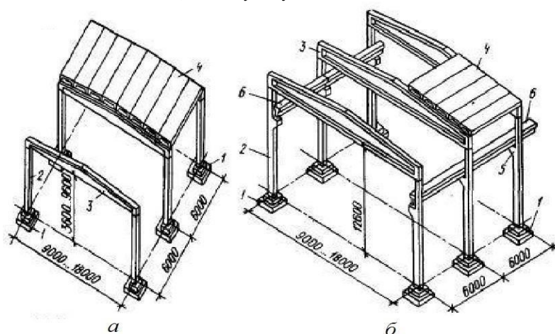
Рис. 112. Конструктивные схемы унифицированных зданий систем водоснабжения и канализации 9...18 м:
