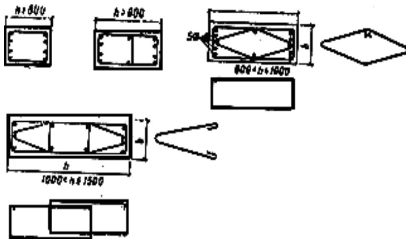
Рис. 69. Армирование внецентренно-сжатых колоннпрямоугольного сечения
