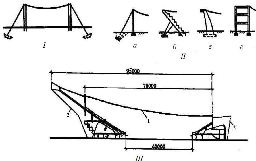
Рис. 53. Висячие покрытия:
