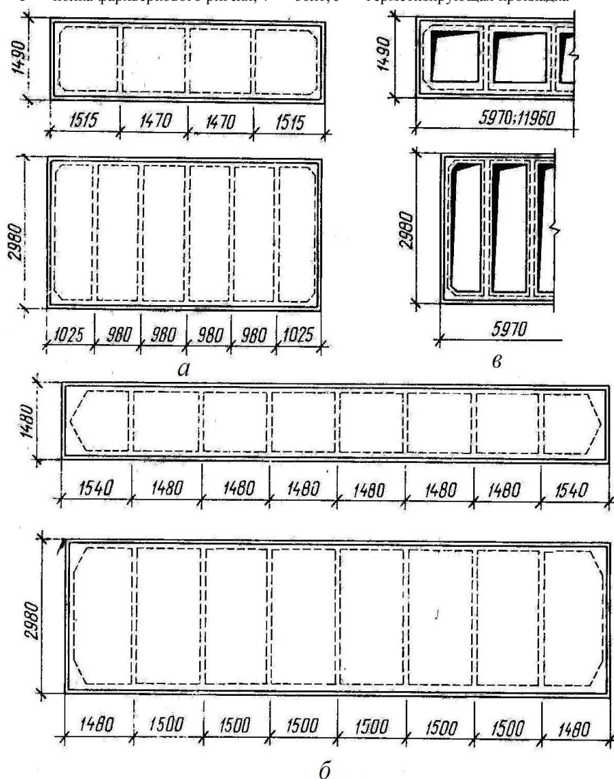
Рис. 107. Железобетонные ребристые панели покрытия промышленных зданий:
