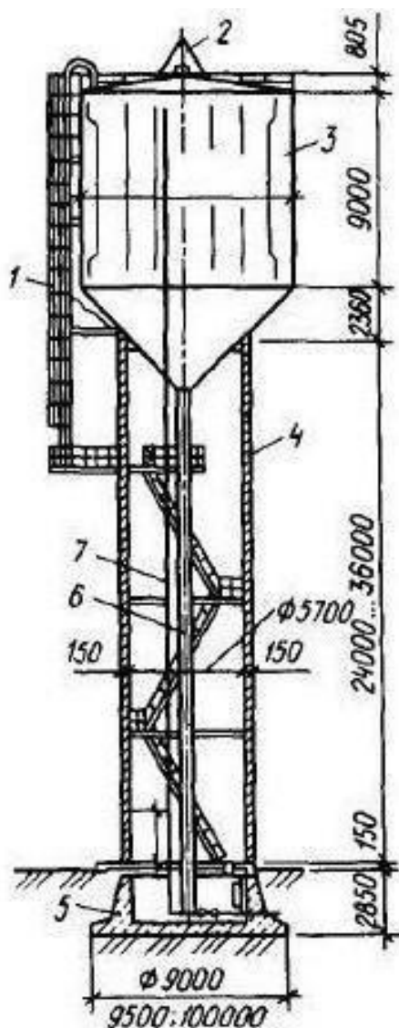
Рис. 114. Типовая водонапорная башня с цилиндрической опорой из монолитного железобетона: 1 — лестница; 2 — молниеотвод; 3 — резервуар; 4 — опора; 5 — фундамент; 6 — напорно-разводящий стояк; 7 — напорно-разводящая труба
