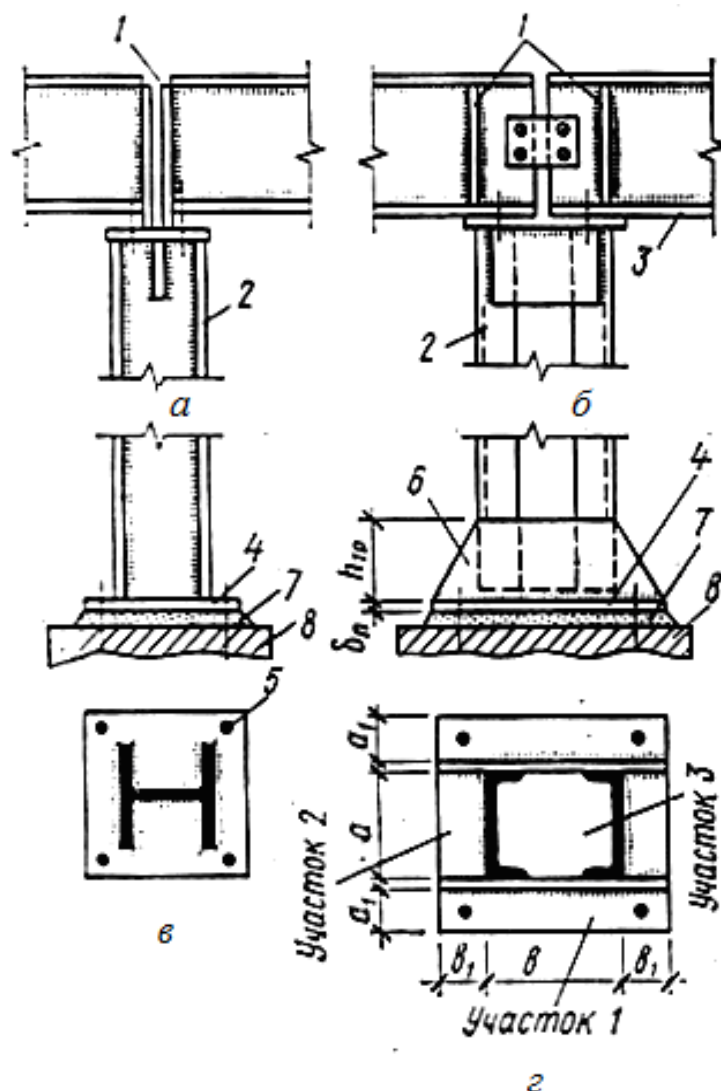
Рис. 62. Конструкция оголовков и баз колонн: а — оголовок с передачей нагрузки через торцевые ребра; б — то же, через ребра, расположенные над полками колоннами; в — база из одного опорного листа; г — база с трассерами; 1 — опорные ребра; 2 — колонна; 3 — балка; 4 — опорная плита; 5 — анкерные болты; 6 — трассера; 7 — выравнивающий слой мелкозернистого бетона или раствора; 8 — фундамент
