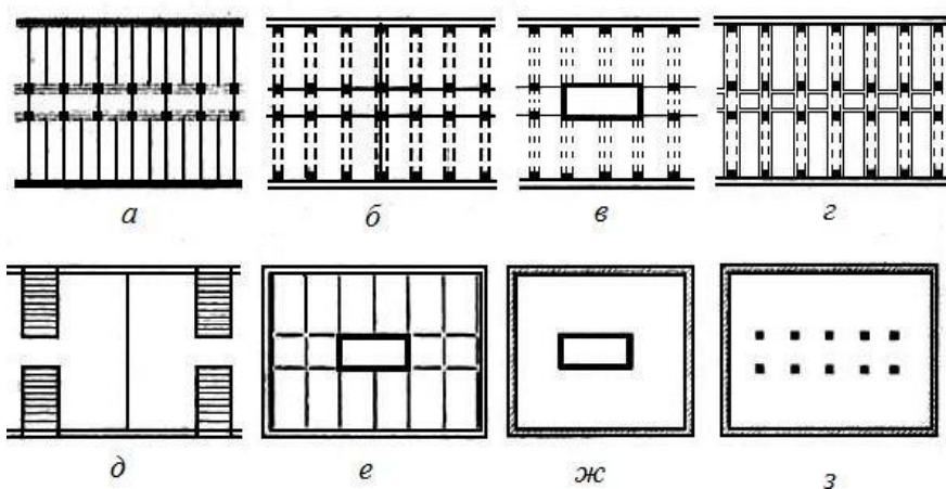
Рис. 5. Комбинированные конструктивные системы: а — с неполным каркасом; б — каркасно-диафрагмовая; в — каркасно-ствольная; г — каркасно-блочная; д — блочно-стеновая; е — ствольно-стеновая; ж — оболочково-ствольная; з — каркасно-оболочковая
