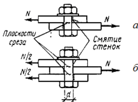
Рис. 57. Болтовые соединения:
