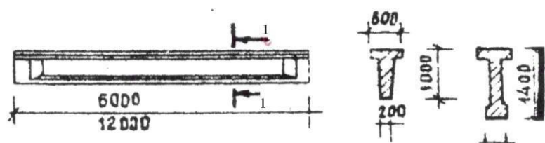
Рис. 92. Железобетонные подкрановые балки
