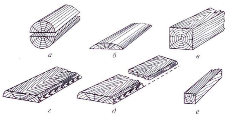
Рис. 74. Основные виды пиломатериалов: а — пластины; б — горбыль; в — брус; г — необрезная доска (с обзолом); д — обрезная доска; е — брусок
