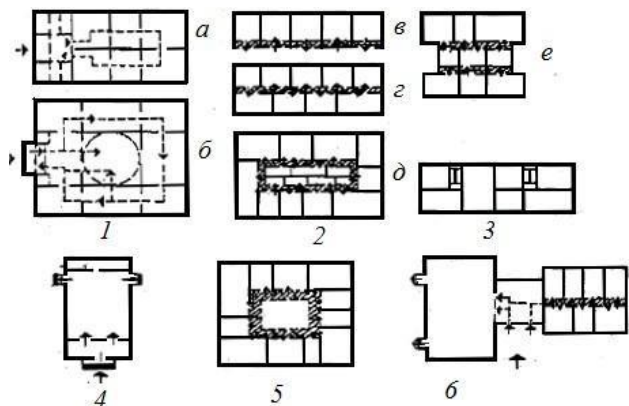
Рис. 3. Объемно-планировочные структуры общественных зданий: 1 — анфиладная; 2 — с горизонтальными коммуникациями; 3 — секционная; 4 — зальная; 5 — атриумная (с внутренним двориком); 6 — комбинированная; а — анфиладная линейная; б — то же центрическая; в — галерейная; г — коридорная; д — коридорно-кольцевая; е — двухкоридорная
