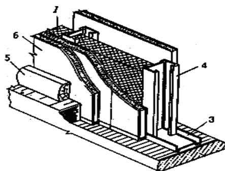
Рис. 46. Перегородки из листовых материалов на металлическом каркасе из гнутых профилей:
