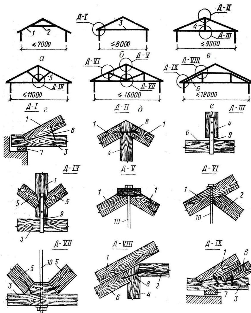
Рис. 81. Висячие стропила — конструктивные схемы и детали узлов: а, б — по схеме треугольной арки; в, г, д, е — по схеме фермы; 1 — стропильная нога; 2 — ригель; 3 — затяжка; 4 — стойка (бабка); 5 — подкос; 6 — нарожник; 7 — мауэрлат; 8 — металлическая скоба; 9 — металлический хомут; 10 — металлическая подвеска
