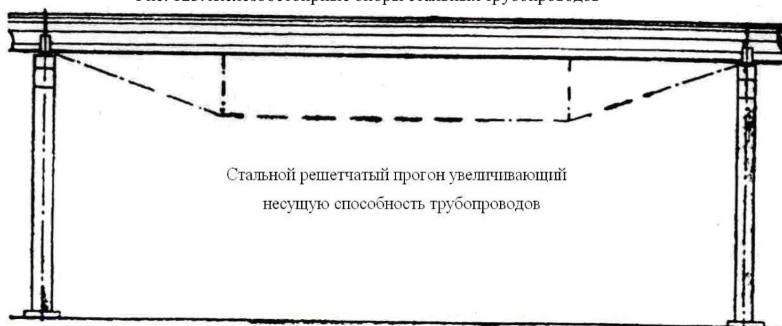
Рис. 123. Железобетонные опоры стальных трубопроводов
