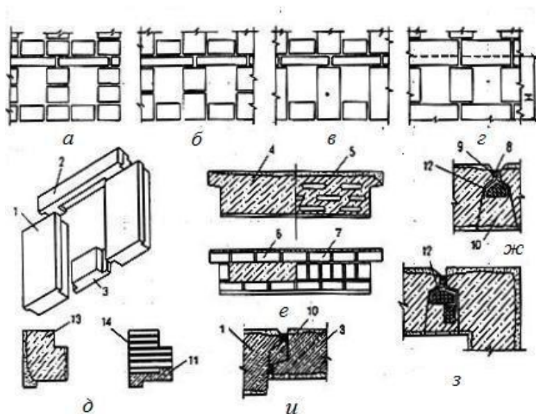
Рис. 17. Крупноблочные стены:
