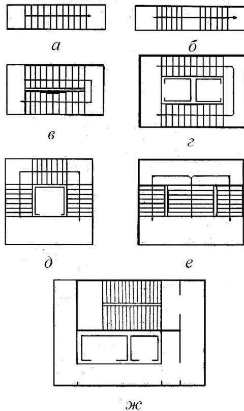
Рис. 26. Основные геометрические схемы лестниц:
