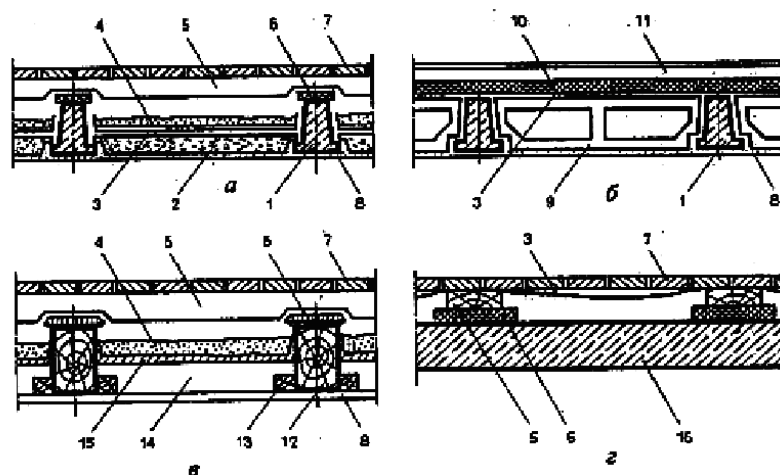
Рис. 34. Варианты конструкции междуэтажного перекрытия:
