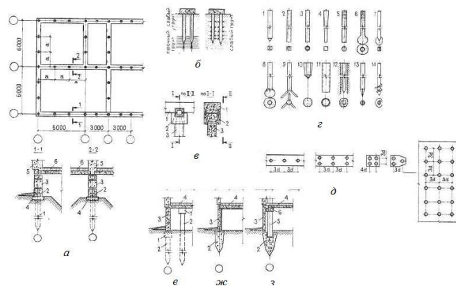
Рис. 11. Свайные фундаменты
