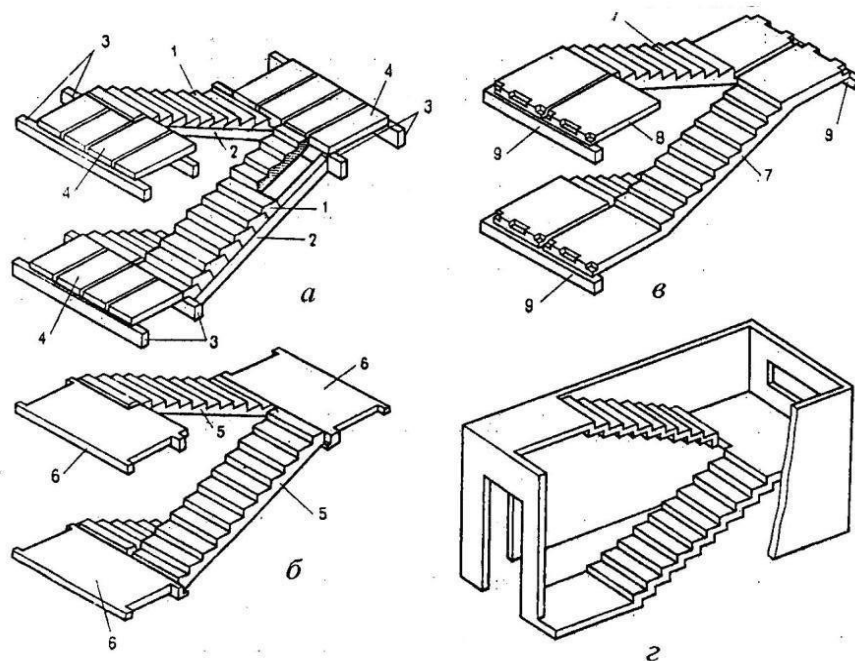
Рис. 27. Варианты разрезки сборных лестниц:
