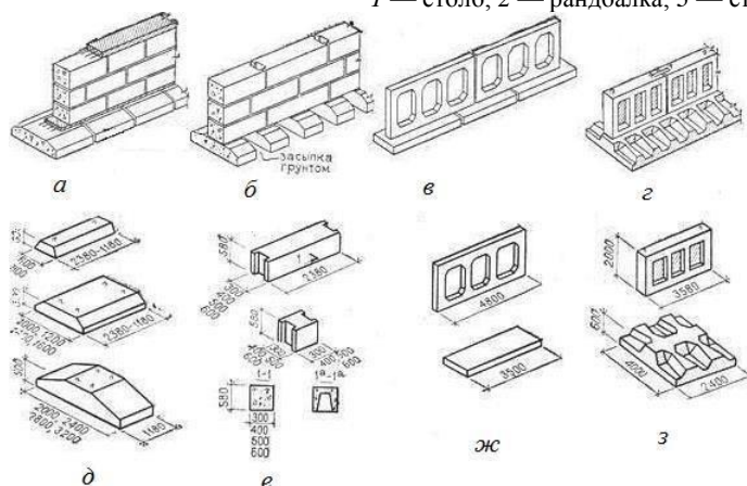
Рис. 10. Сборные бетонные и железобетонные ленточные фундаменты:
