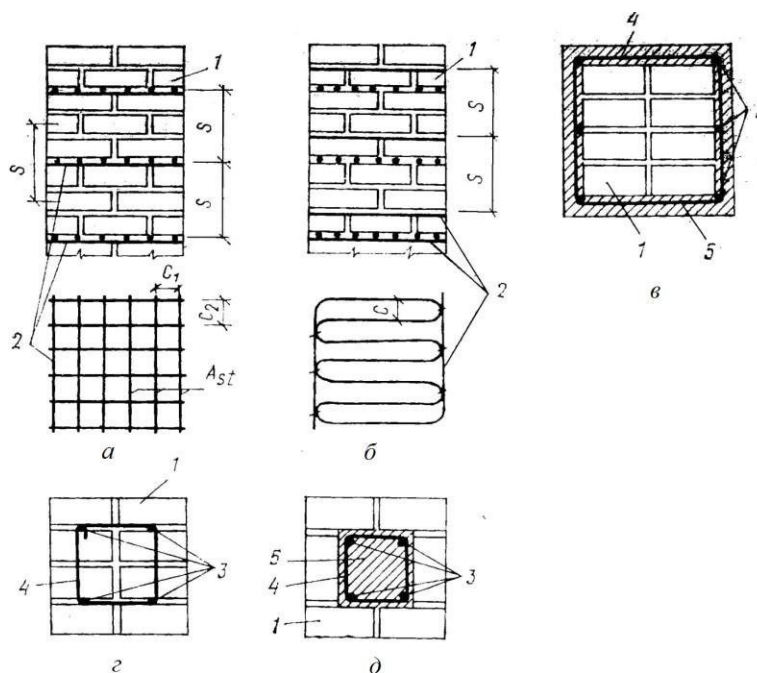
Рис. 85. Армокаменные конструкции:
