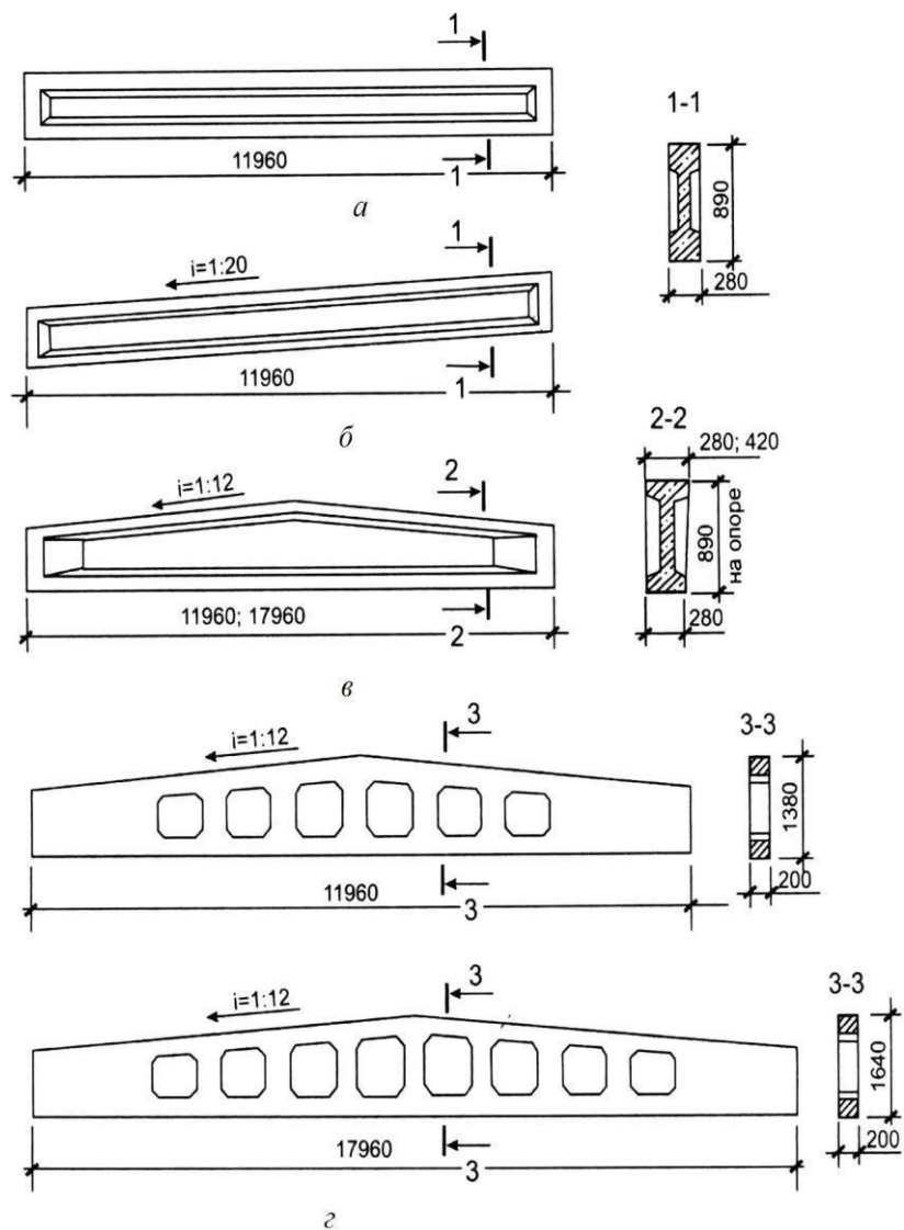
Рис. 72. Железобетонные балки покрытия: a — балка с параллельными поясами; б — односкатная балка таврового сечения; в — то же для двускатных покрытий; г — решетчатая балка для двускатных покрытий (перфорированная балка)
