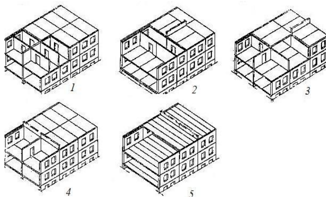
Рис. 7. Конструктивные схемы бескаркасных зданий
