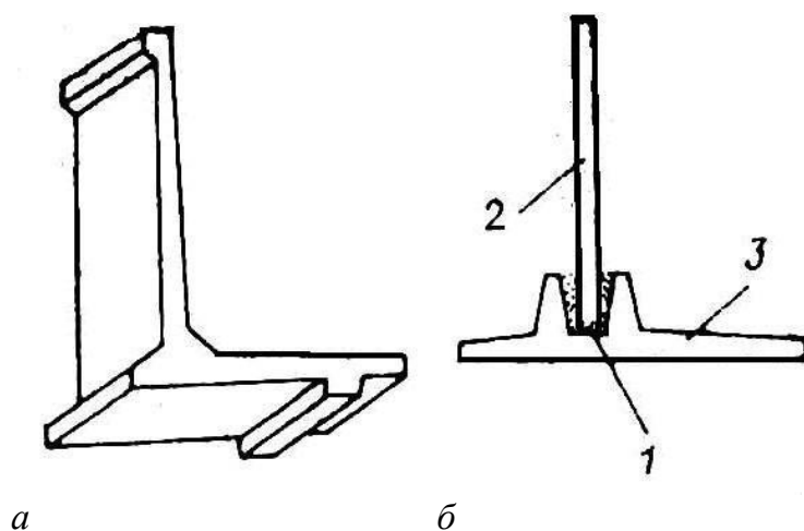
Рис. 121. Сборные подпорные стены углового профиля: а — из элементов углового типа (аксонометрия); б — из плоских элементов; 1 — замоноличиваемый стык; 2 — лицевая плита; 3 — фундаментная плита
