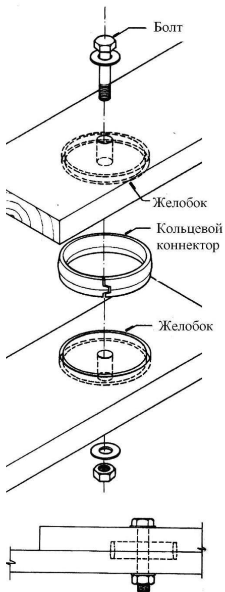
Рис. 78. Принцип соединения деревянных элементов при помощи кольцевых коннекторов
