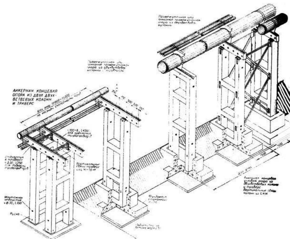
Рис. 125. Общий вид несущих опорных конструкций надземного трубопровода
