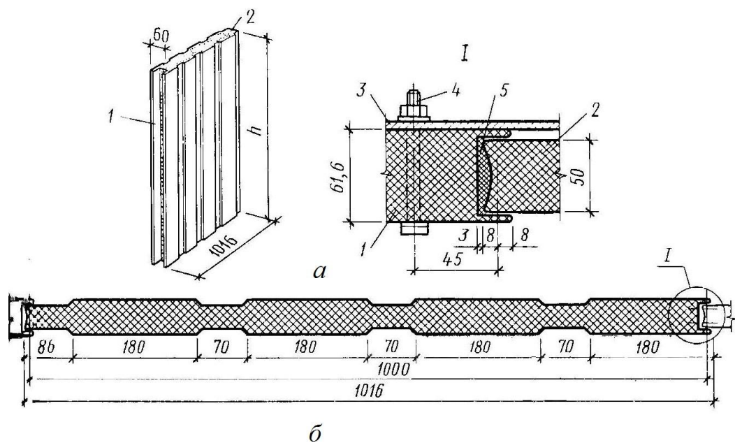
Рис. 106. Металлические панели типа «сэндвич» для стен промышленных зданий:
