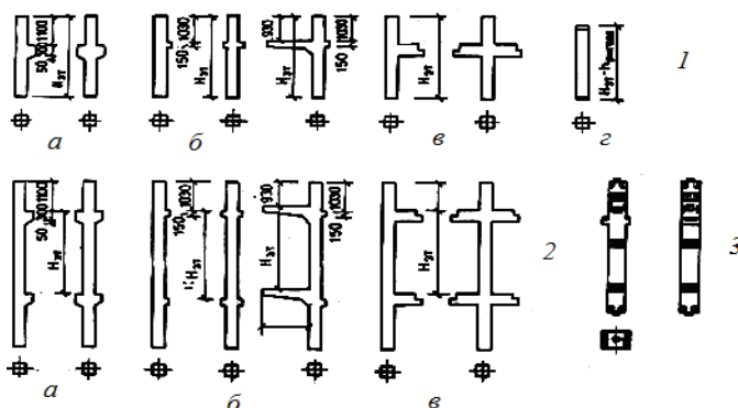
Рис. 22. Колонны каркасов:
