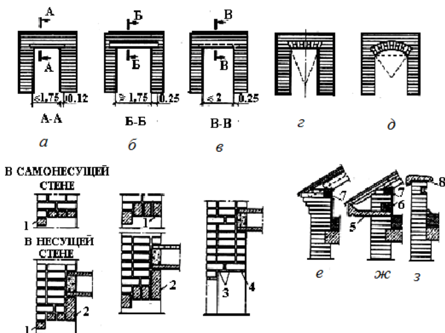
Рис. 16.. Детали каменных стен:
