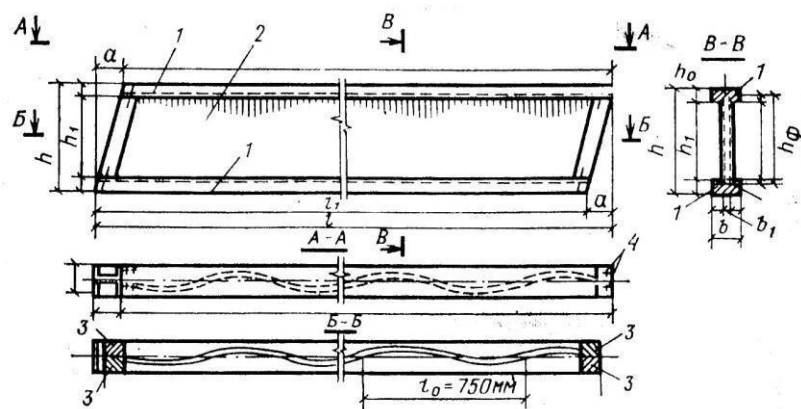
Рис. 83. Деревянная клееная балка с волокнистой фанерной стенкой: 1 — дощатые или брусчатые верхний и нижний пояса; 2 — волнистая фанерная стенка; 3 — дощатые или брусчатые концевые элементы жесткости
