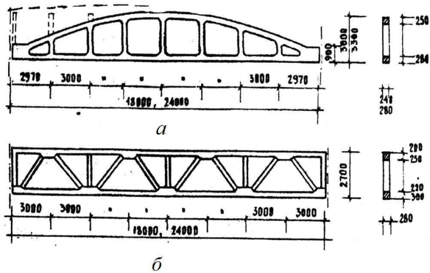
Рис. 94. Стропильные железобетонные фермы: a — сегментная безраскосная ферма; б — ферма с параллельными поясами
