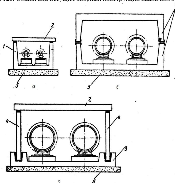
Рис. 125. Общий вид несущих опорных конструкций надземного трубопровода
