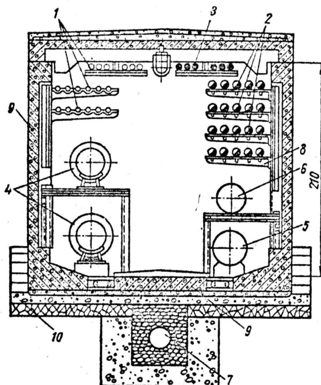
Рис. 128. Размещение подземных сетей в общем коллекторе(проходном канале): 1 — кабели связи; 2 — кабели силовые; 3 — кабели внутреннего обслуживания коллектора; 4 — трубопроводы тепловой сети; 5 — водопровод; 6 — канализация; 7 — дренажная труба; 8 — металлические полочки; 9 — железобетонные блоки; 10 — бетонная подготовка
