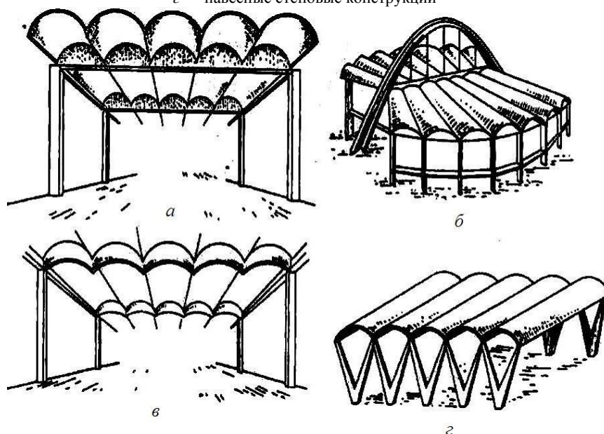
Рис. 52. Многоволновые оболочки:
