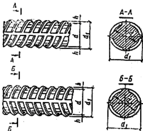
Рис. 66. Горячекатаная арматурная сталь периодического профиля
