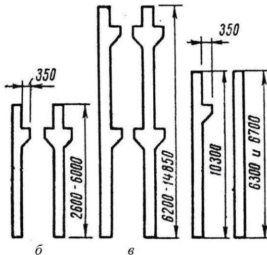
Рис. 102. Железобетонные колонны многоэтажных промзданий: a — для верхних и средних этажей; б — для верхний, средних и нижних этажей; в — для верхних «крановых» этажей
