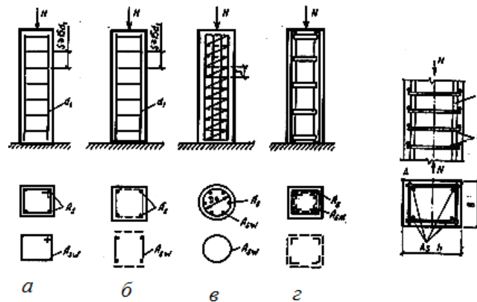
Рис. 67. Центально-сжатые колонны: a — с вязанными каркасами; b — со сварным каркасами; c — со спиралью или сварными кольцами; d — с жесткой арматурой; 1 — продольная арматура; 2 — хомуты
