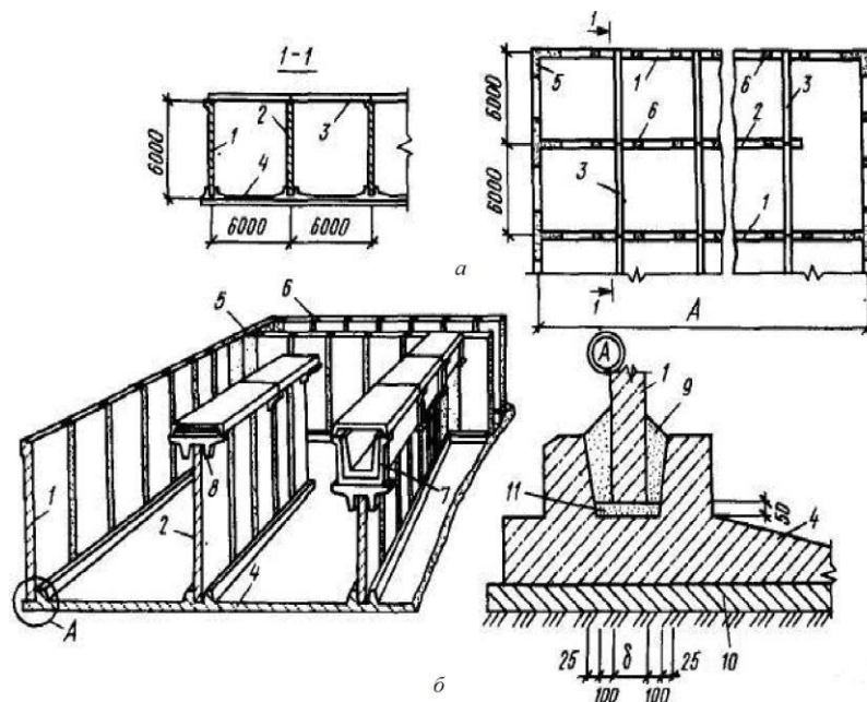
Рис. 117. Конструктивное решение азротенка из железобетонных панелей:
