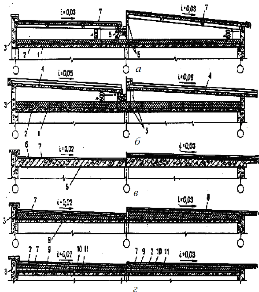
Рис. 33. Конструкции бесчердачных крыш:
