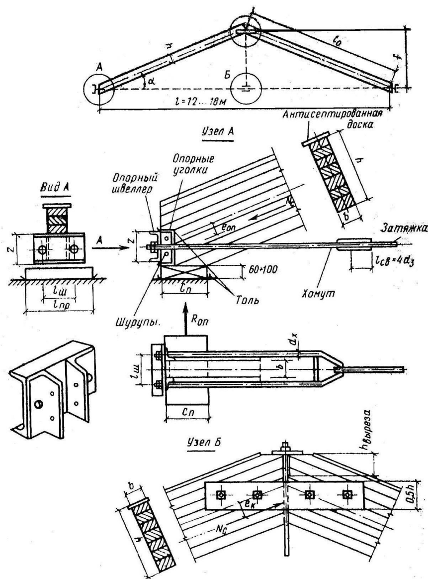
Рис. 84. Трехшарнирная арка треугольного очертания
