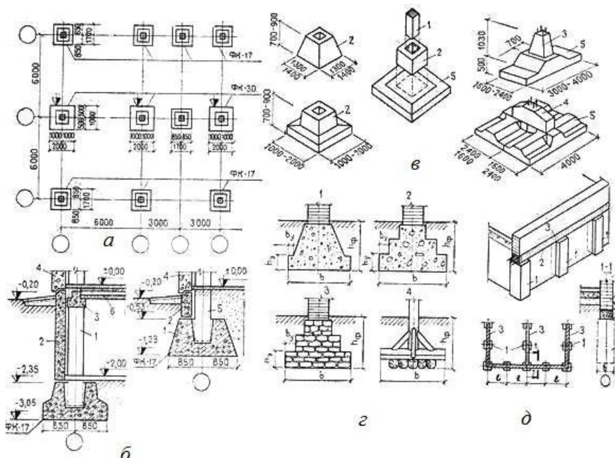
Рис. 9. Отдельно стоящие фундаменты:
