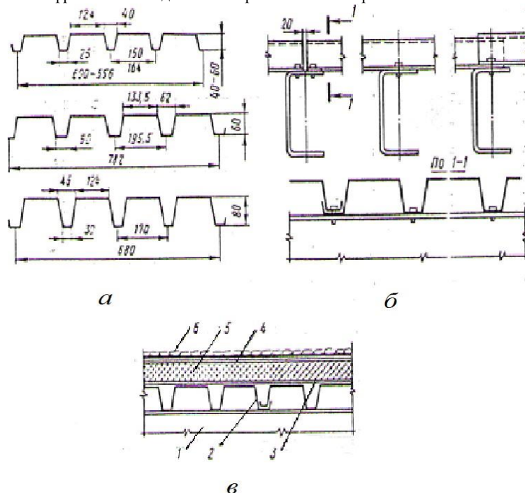
Рис. 108. Покрытия из стального профилированного настила: a — типы настилов; б — варианты крепления настилов; в — утепленное покрытие; 1 — прогон; 2 — настил; 3 — слой рубероида на мастике; 4 — основной кровельный ковер; 5 — пенополистирол; б — гравий, втопленный в мастику
