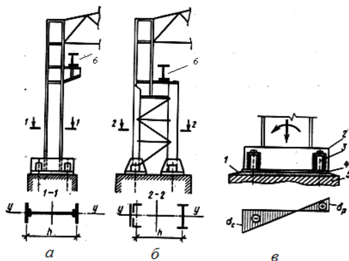
Рис. 63. Внецентренно-сжатые колонны:
