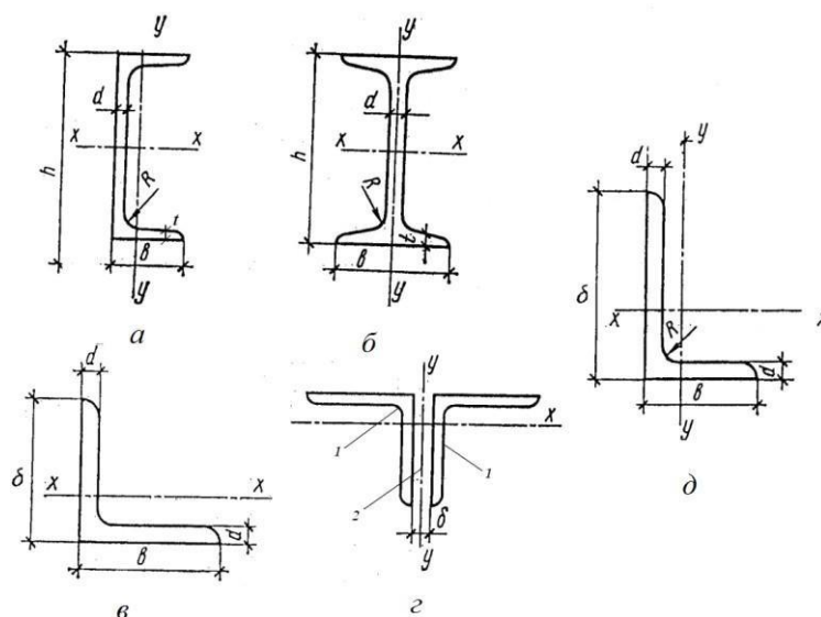
Рис. 55. Основные виды прокатных профилей:
