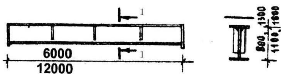
Рис. 96. Металлические стропильные фермы: a — ферма с параллельными поясами из прокатных уголков или широкополочных тавров; б — ферма с перекрестной решеткой из прокатных уголков или трубчатых элементов
