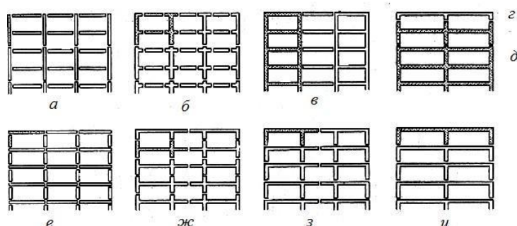
Рис. 21. Способы членения каркаса на элементы:
