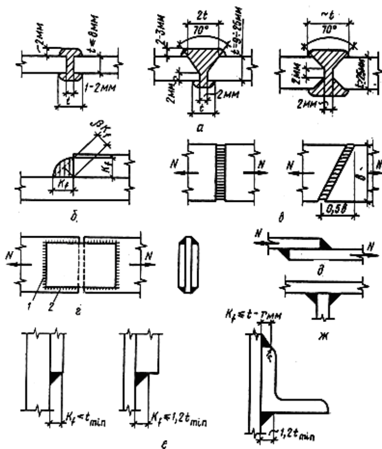
Рис. 56. Типы сварных швов и соединений:
