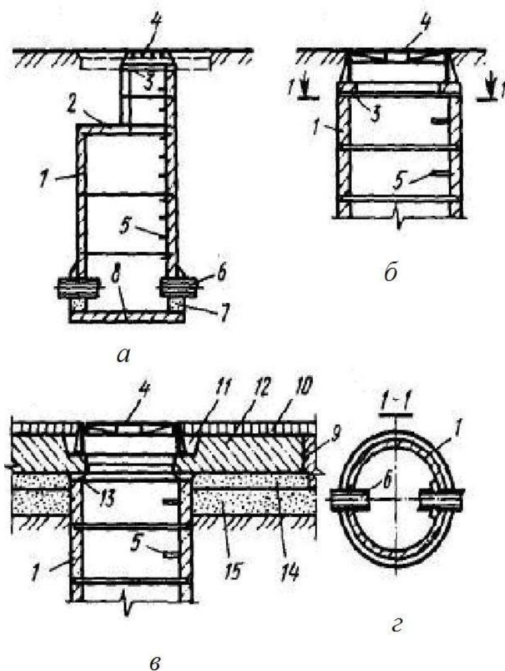
Рис. 122. Конструкция смотрового колодца систем водоснабжения и водоотведения:
