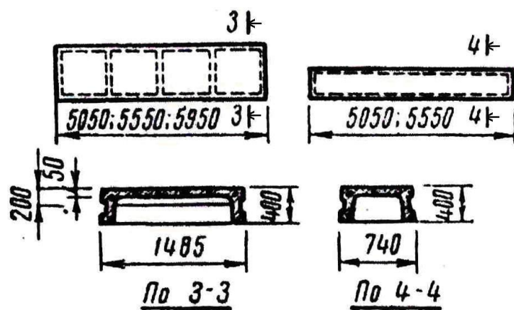
Рис. 104. Сборные железобетонные плиты перекрытий многоэтажных промышленных зданий
