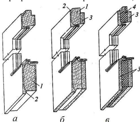
Рис. 18. Бетонные панели наружных стен:
