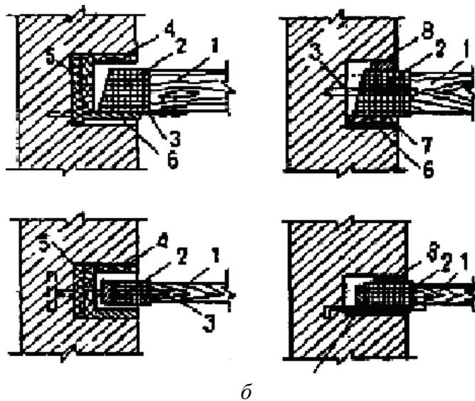
Рис. 37. Опираие деревянных балок на каменные стены: a — при утепленном гнезде; б — глухая заделка гнезда; 1 — балка; 2 — обертка толемна мастике; 3 — анкер стальной; 4 — дощатый короб; 5 — термовкладыш; б — два слоя толя; 7 — антисептированная подмазка; 8 — заделка раствором
