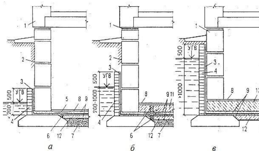
Рис. 13. Гидроизоляция фундаментов: а — при напоре грунтовых вод менее 200 мм; б — при напоре 200-1000 мм; в — при напоре свыше 1000 мм; 1 — рулонная гидроизоляция; 2 — окрасочная гидроизоляция (промазка горячим битумом за 2 раза); 3 — оклеечная гидроизоляция; 4 — защитная стенка из кирпича; 5 — стеклоткань; 6 — деформационный шов; 7 — глина; 8 — пол подвала; 9 — стяжка; 10 — железобетонная плита; 11 — пригрузочный слой из бетона; 12 — подготовка
