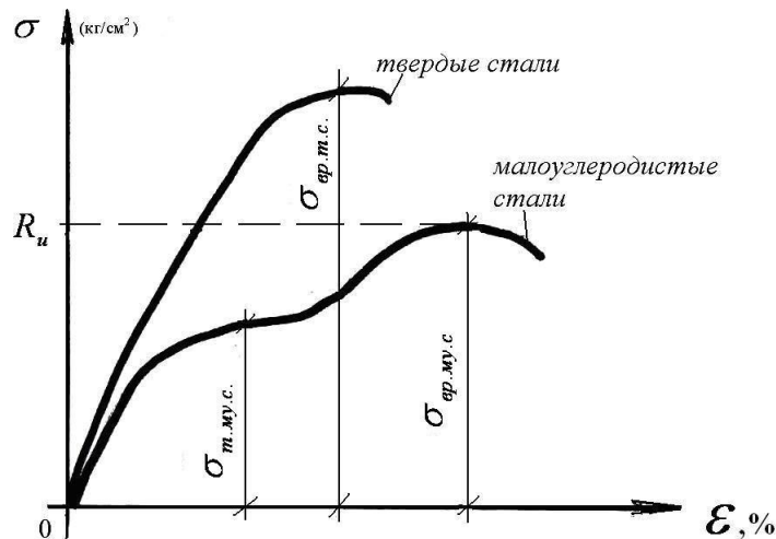
Рис. 54. Схематическая диаграмма зависимости между напряжениями для различных классов сталей
