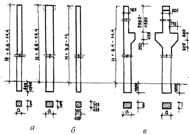
Рис. 90. Сборные железобетонные колонны каркаса: а — железобетонные колонны для бескрановых зданий; б — железобетонные колонны фахверка; в — железобетонные колонны для зданий смостовыми кранами средней грузоподъемности
