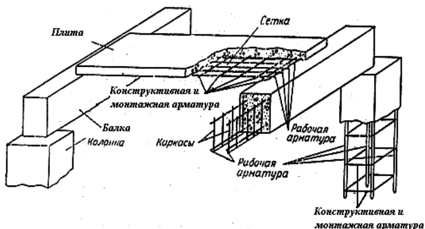
Рис. 65. Способ армирования железобетонных элементов каркасами и сетками
