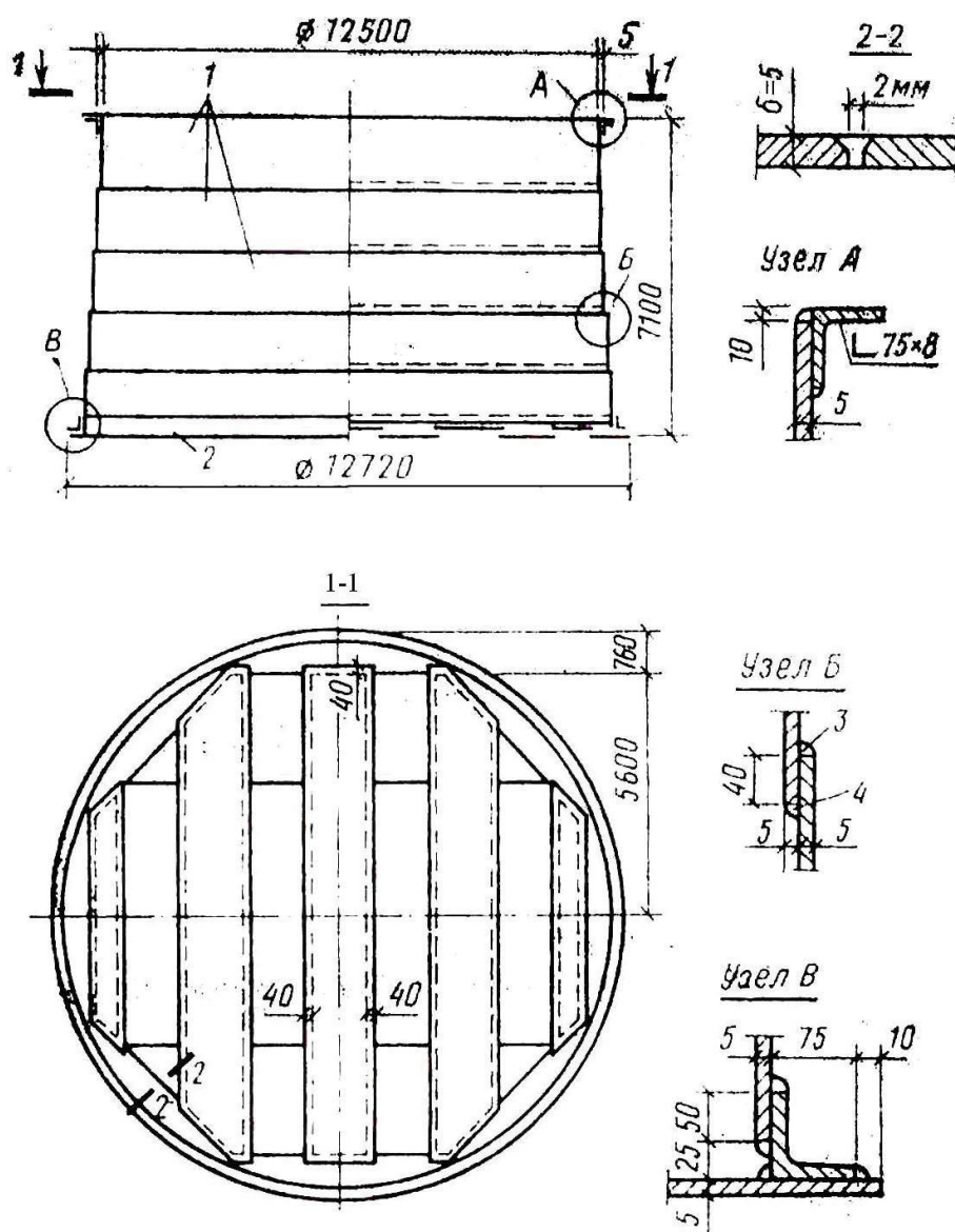
Рис. 116. Стальной резервуар с плоским дном: 1 — пояса стенки; 2 — днище; 3 — сплошной шов; 4 — прерывистый шов
