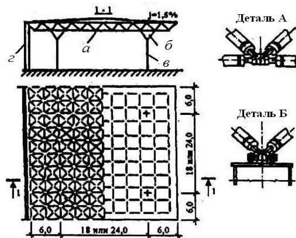
Рис. 51. Перекрестно-стержневые покрытия («структуры»).
