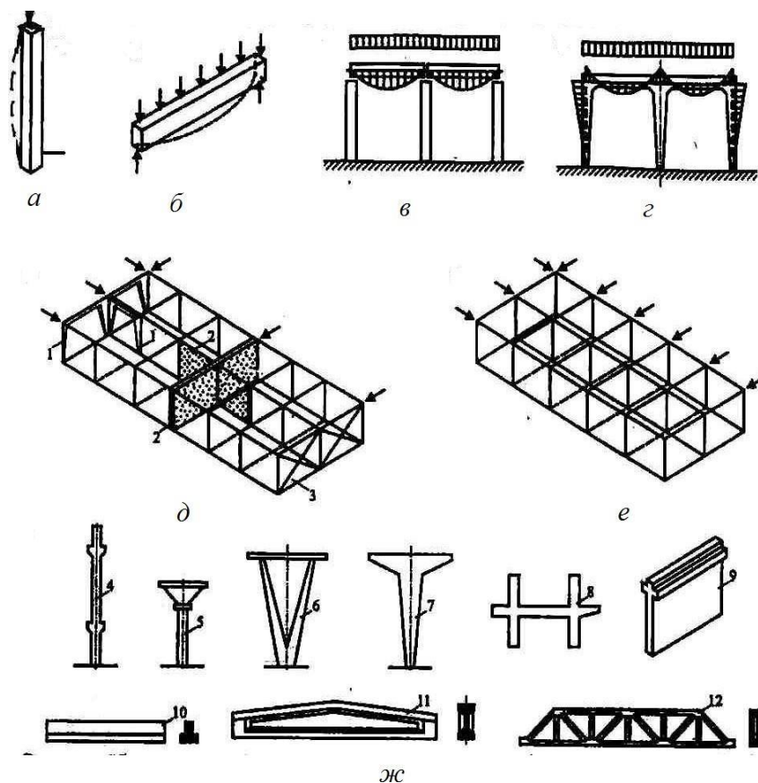
Рис. 48. Стоечно — балочные несущие конструкции:
