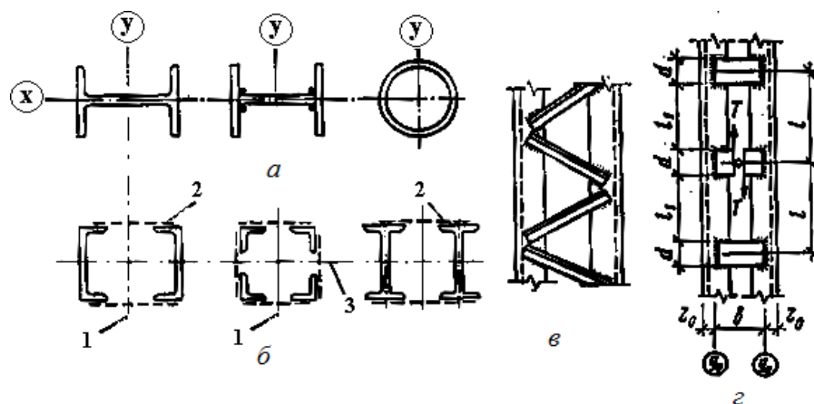
Рис. 61. Центально-сжатые колонны: а — сечения сплошных колонн; б — сечения сквозных колонн; в — решетка колонн из уголков; г — колонная с планками; 1 — свободная ось; 2 — соединительная решетка; 3 — материальная ось
