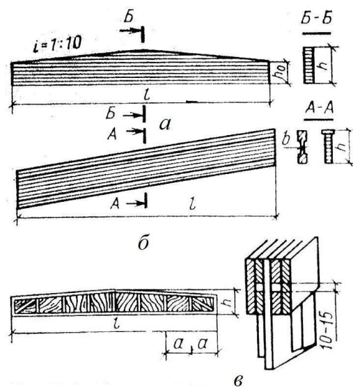
Рис. 82. Клееные балки: а — двускатные прямоугольного сечения; б — с параллельными поясами двутаврового и прямоугольного сечения; в — дощатофанерные двутаврового сечения
