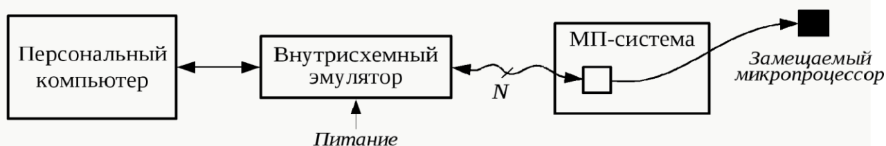
Рисунок 16.2 – Отладка с помощью внутрисхемного эмулятора
