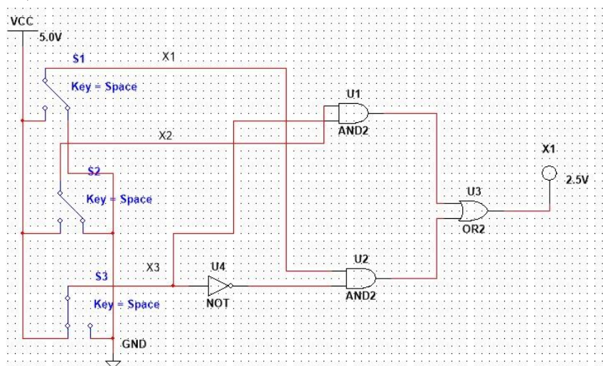
Рисунок 2 - Комбинационная схема
