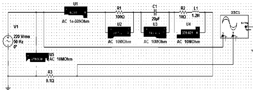
Рис. 3.1 – Схема цепи с последовательным соединением резистора, катушки и конденсатора
