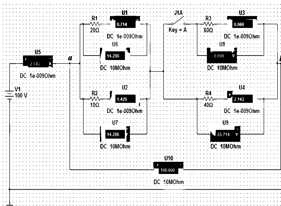
Рисунок 2.1 – Схема цепи
