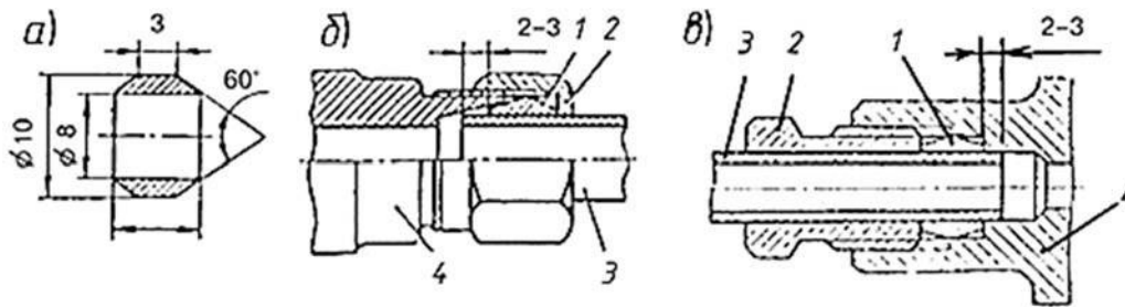
а – конусная муфта; б, в – соединение трубопровода; 1 – конусная муфта (ниппель); 2 – гайка; 3 – трубка; 4 – присоединяемая деталь (штуцер)
