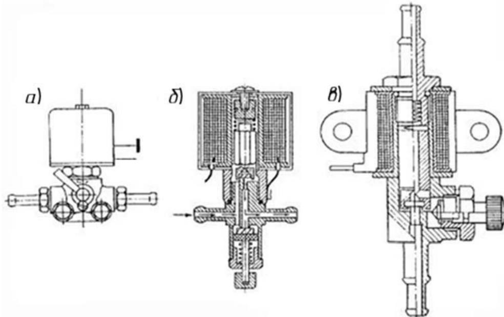
а – с ручкой; б – с нижним вентилем; в – с боковым вентилем
