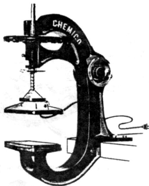
Рис. 14. Настольный электровулканизатор для ремонта камер фирмы «CHEMICO» (Италия)
