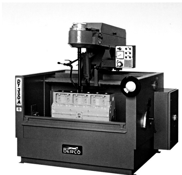
Рис. 2. Хонинговальный станок.
