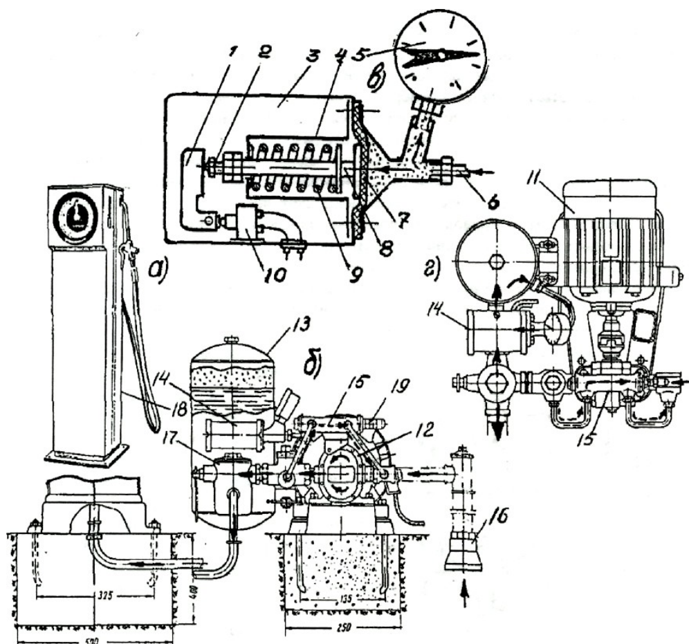
Рис. 3. Установка для раздачи масел для двигателей:
