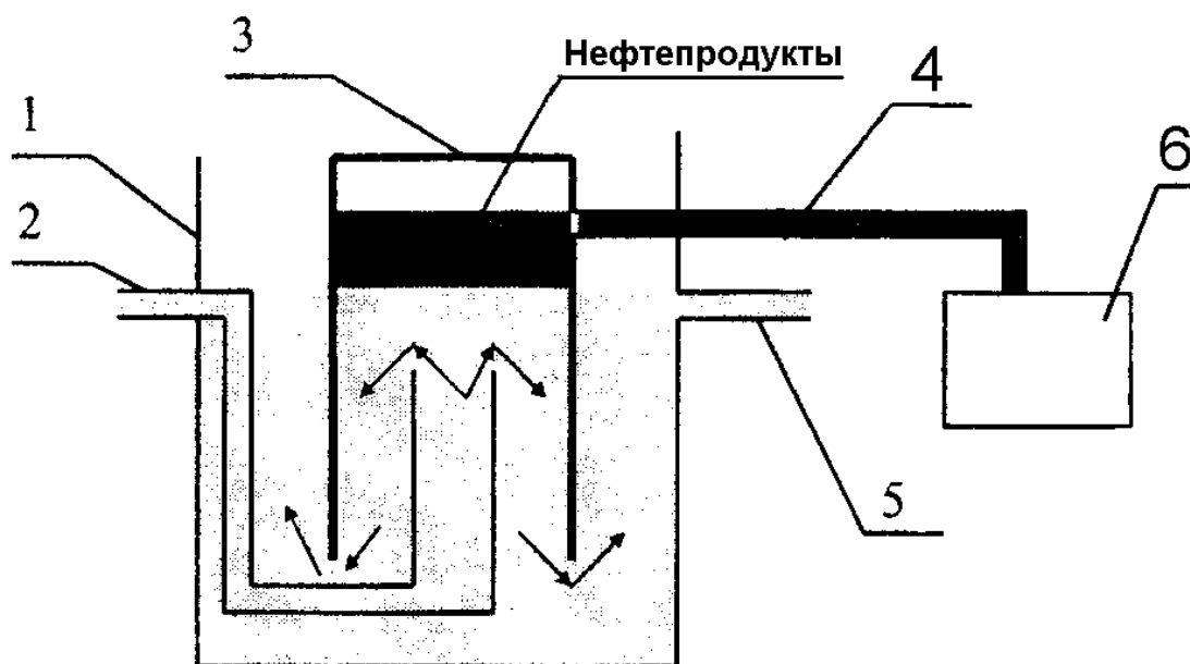
Рисунок 3.2 Схема маслобензоуловителя.
