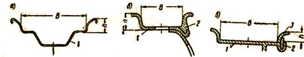
Рис. 1. Ободы колес: В - ширина обода; h - высота закраины; 1 - обод; 2 - съемное разрезное бортовое кольцо, 3 - запорное бортовое кольцо
