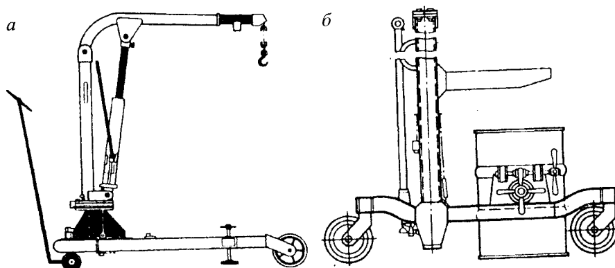
Рисунок 7. Ручная тележка с крановой стрелой (а) и с кантователем для бочек (б)
