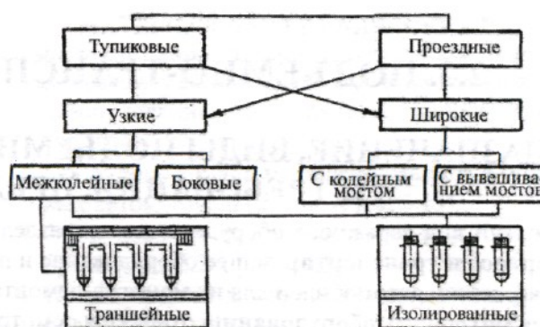
Рис. 5.1. Схема классификации осмотровых канав
