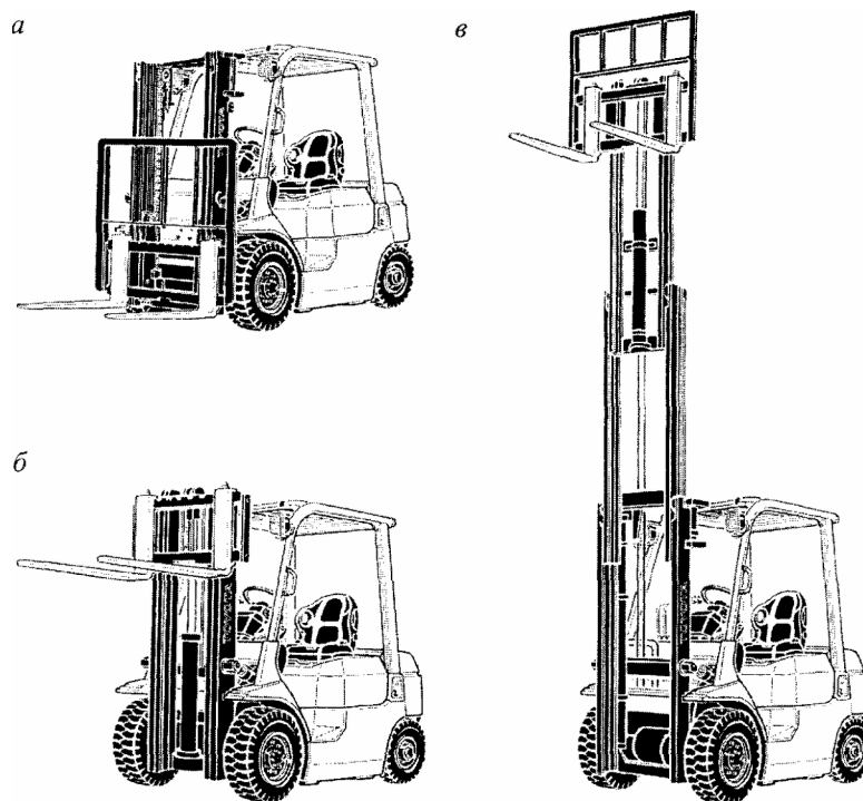
Рисунок 13. Электропогрузчики с различными типами мачт: а-VnSV;б-FV;е-FSV
