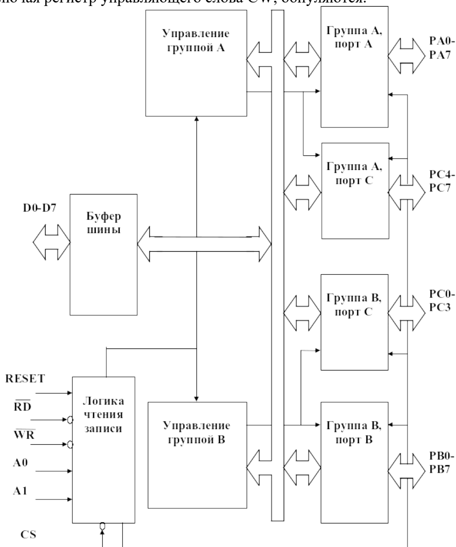
Рис. 1. Структурная схема БИС ППА К580ВВ55А
