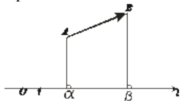
Рис. 10. Проекция вектора на ось
