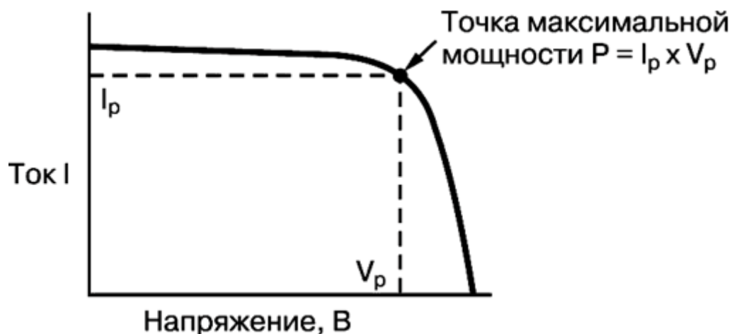
Рисунок 2 – Вольт-амперная характеристика фотоэлемента
