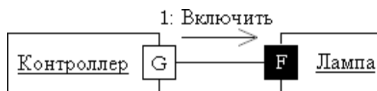
Рисунок 2 – Пример диаграммы Collaboration
