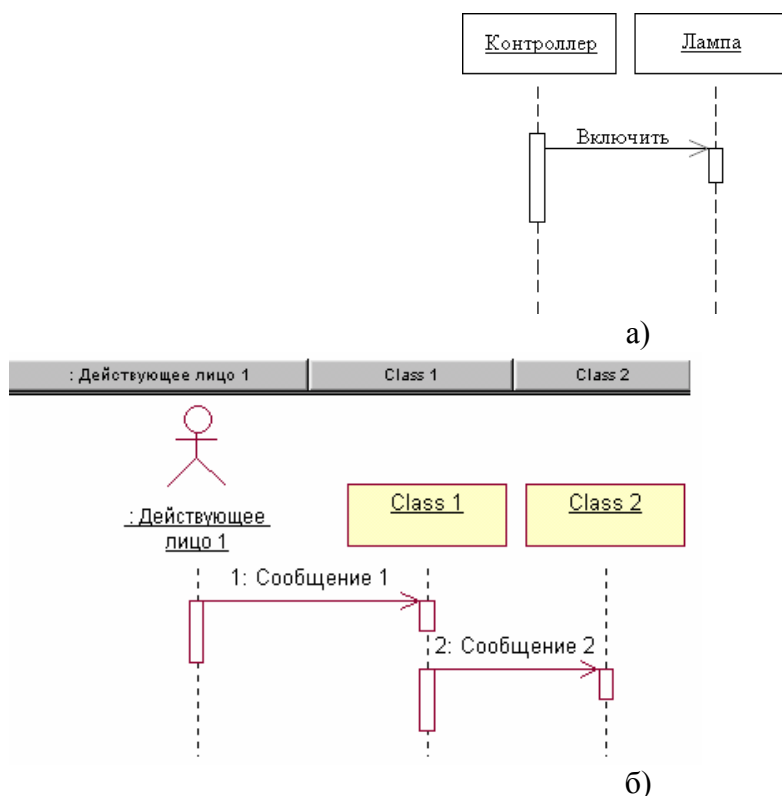
Рисунок 1 – Примеры Sequence диаграмм
