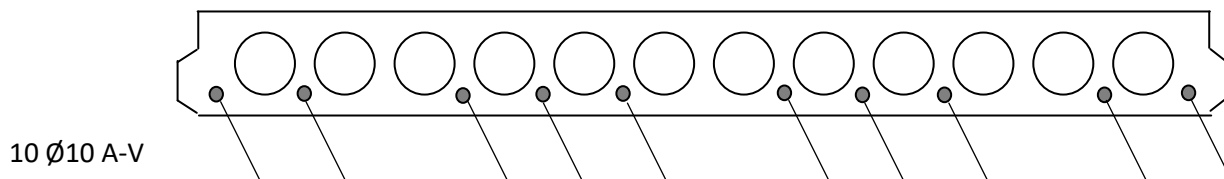
Рисунок 5 - Размещение продольной напрягаемой арматуры в поперечном сечении плиты
